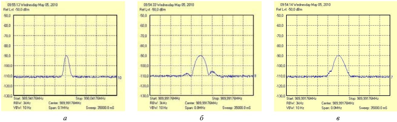
Рис. 3. Рівень сигналу (а), діаграма направленості за азимутом (б) та кутом місця (в) тестової антени
