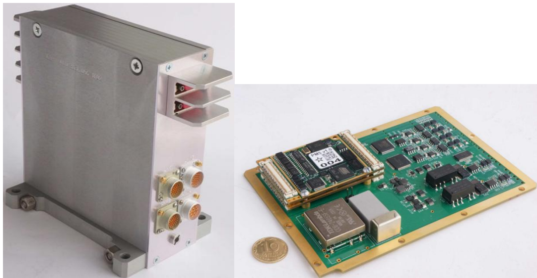
Рис. 4. Зовнішній вигляд центрального блоку та резервованого ПМ
