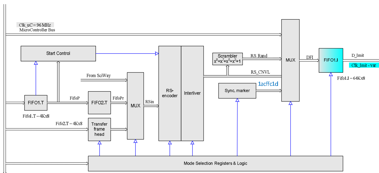
Рис. 1. Кодер Ріда-Соломона
