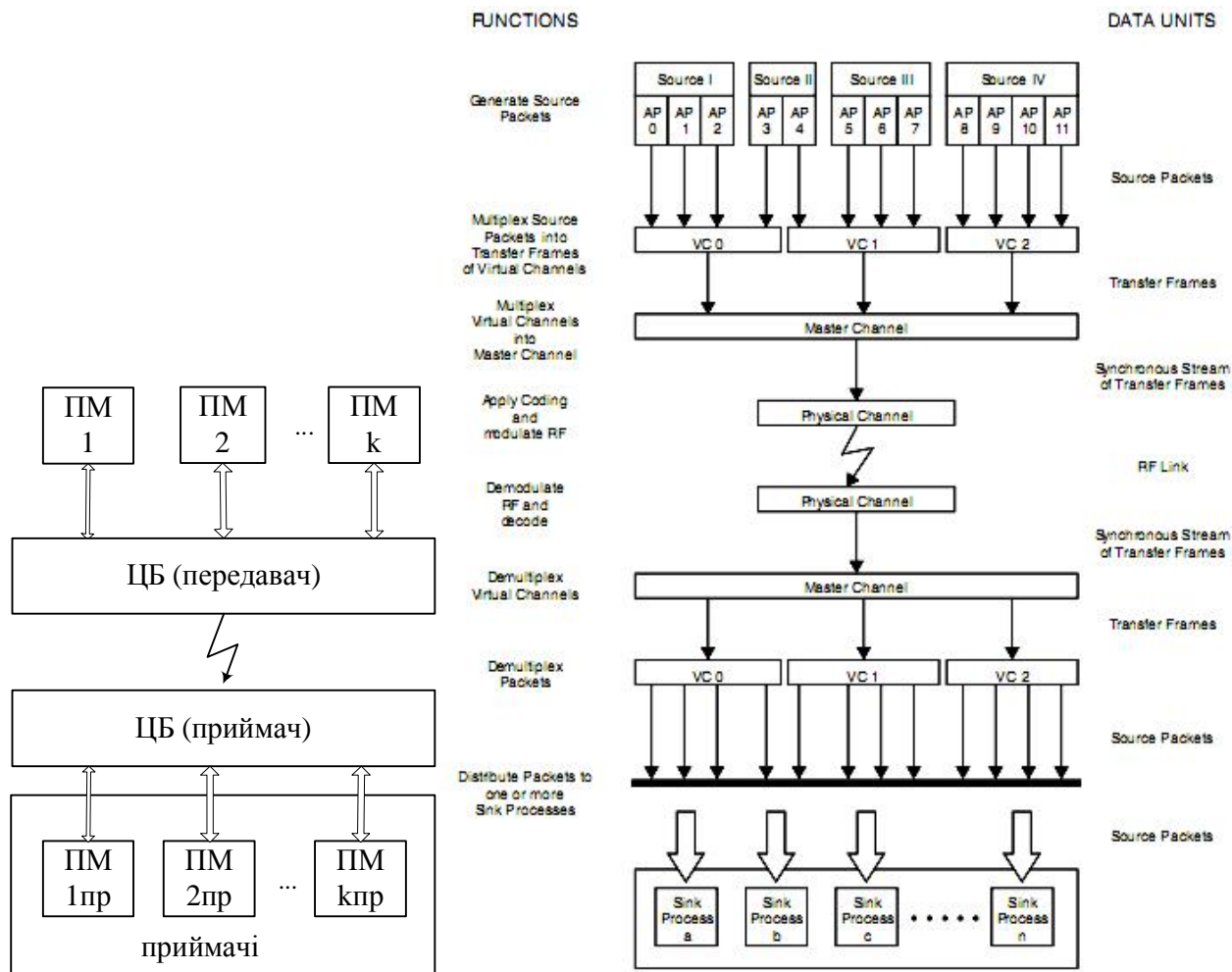
Рис. 6. Модулі СЗНІ в структурі передачі телеметричної інформації
