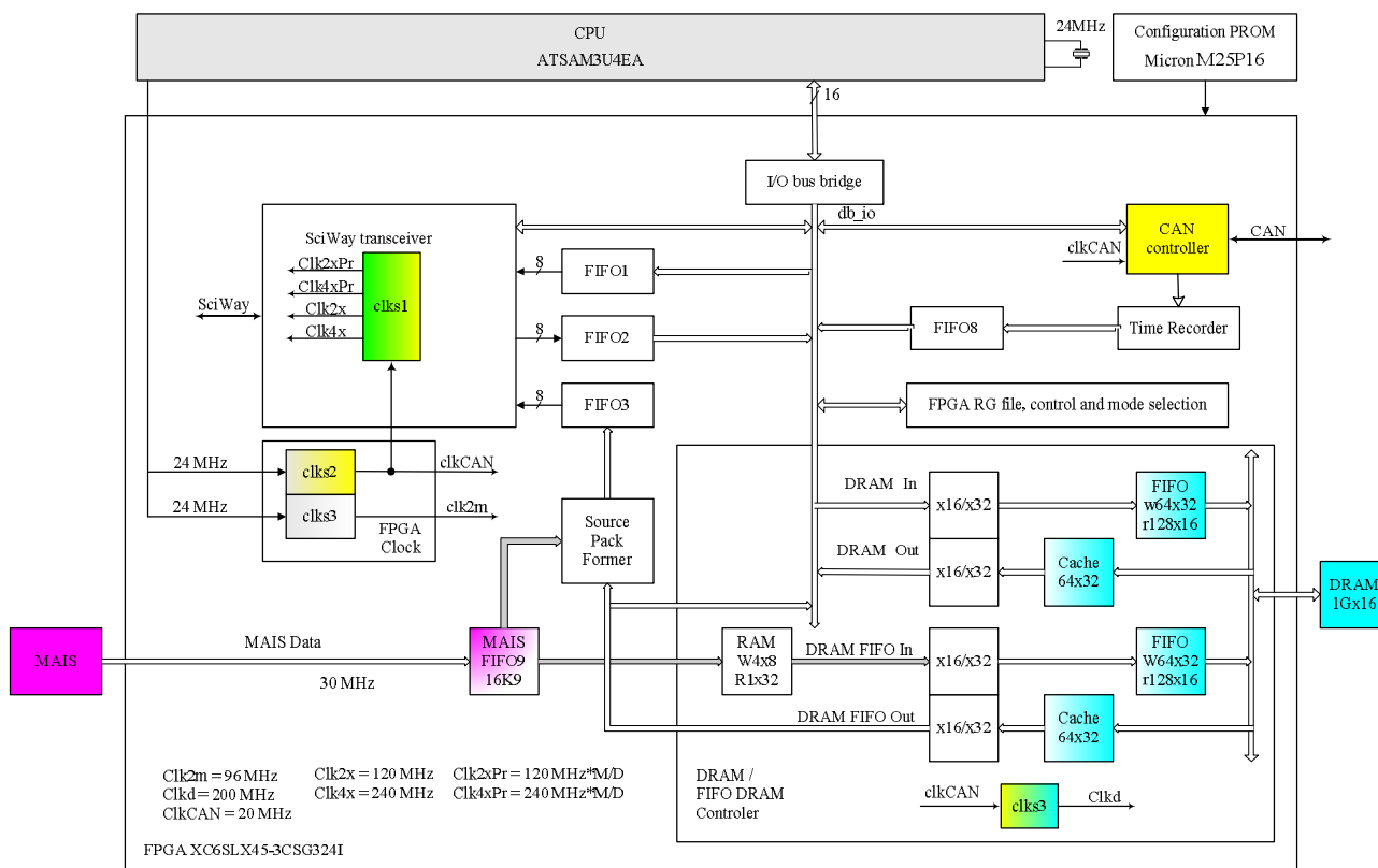
Рис. 3. ПЛІС ПМ MAIC
