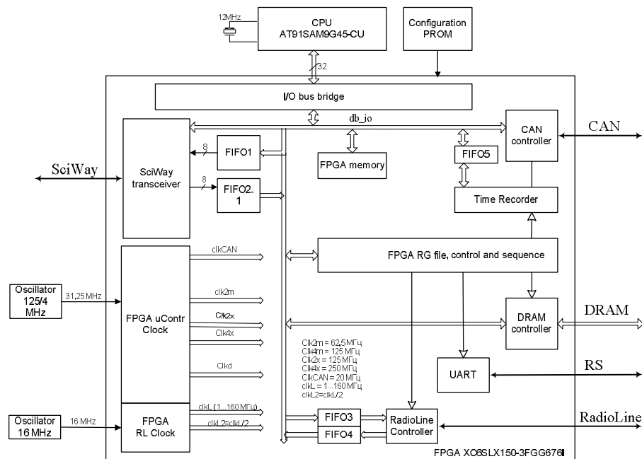
Рис. 5. ПЛІС центрального блоку СЗНІ
