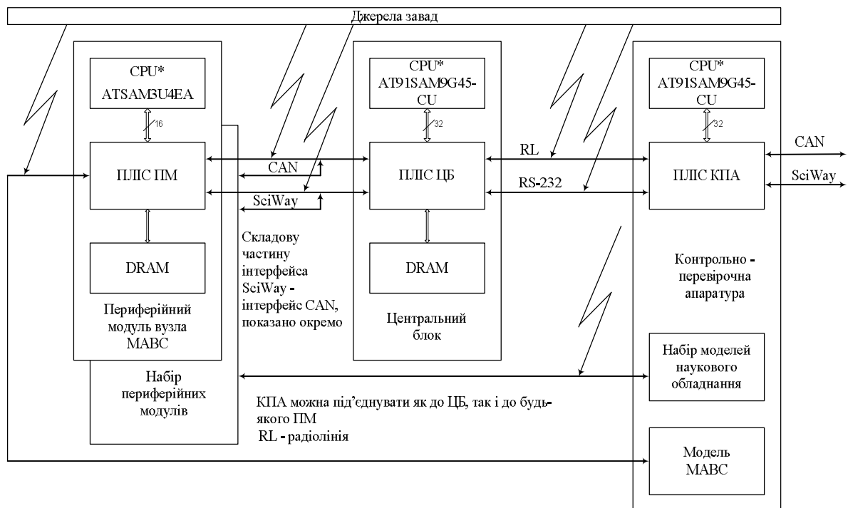
Рис. 8. Модельний стенд КНА «Юносат-мікро»
