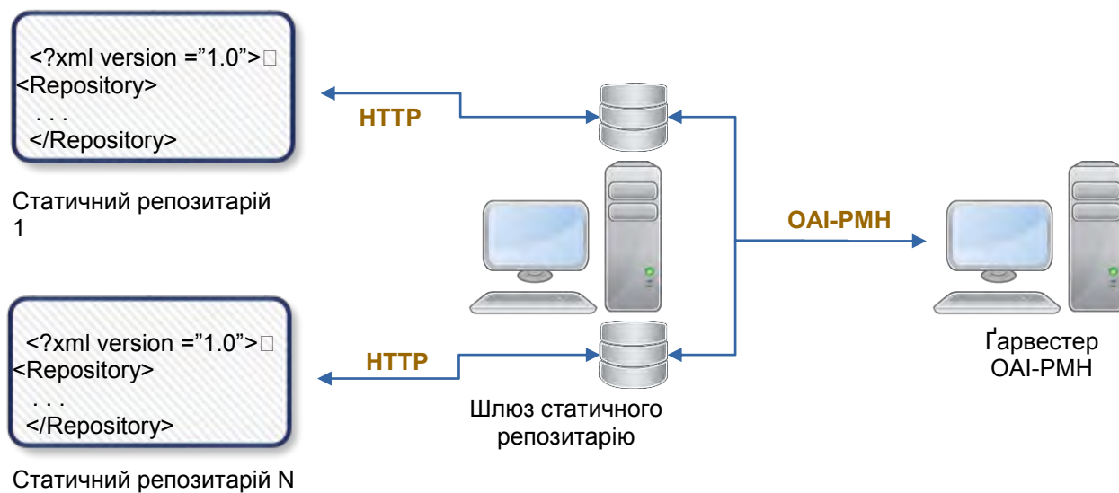
Рис. 2. Взаємодія між статичним репозитарієм, шлюзом та гарвестером.
