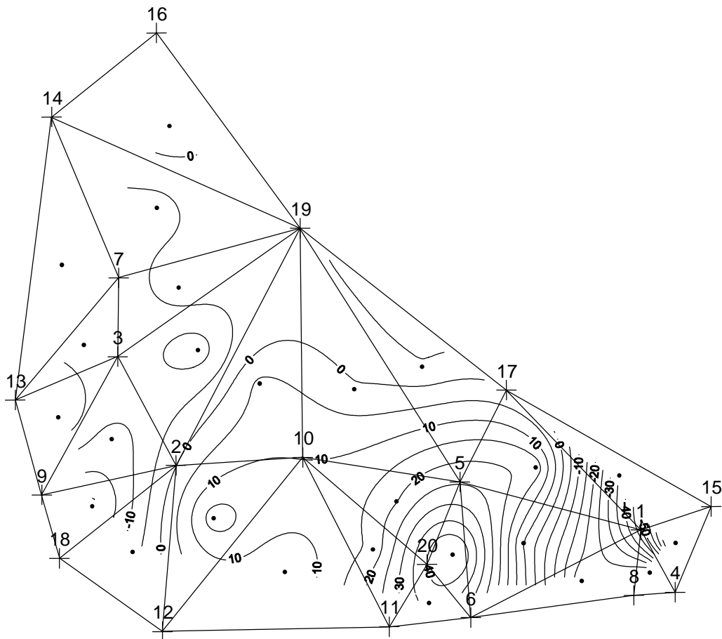
Рис. 2. Розподіл дилатації в одиницях 10^{-7} за результатами вимірів циклів спостережень 1 – 3
