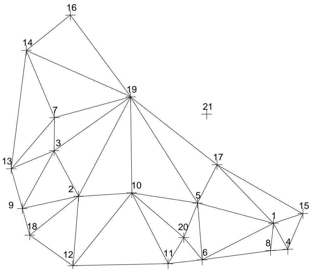
Рис. 1. Схема геодезичної мережі геодинамічного полігона Рівненської АЕС
