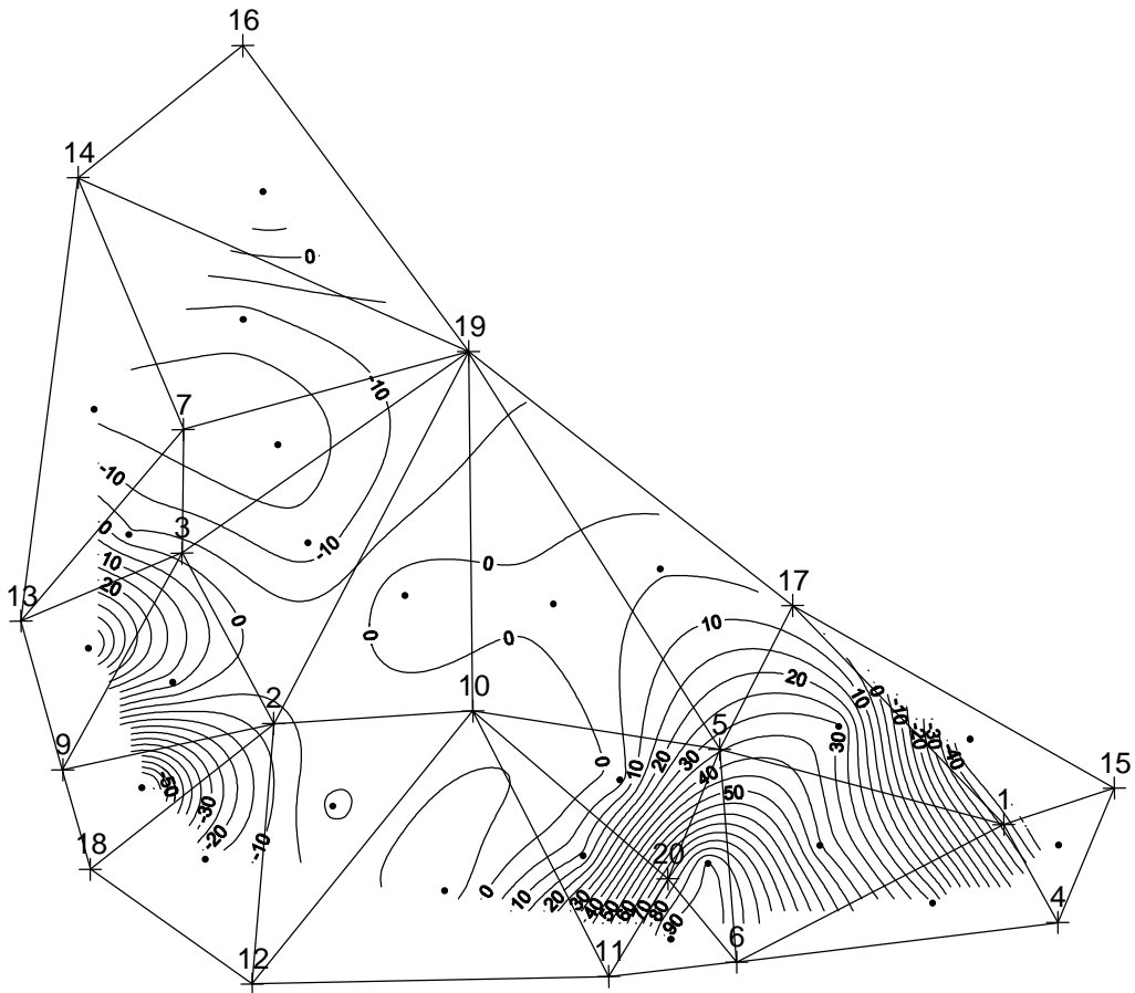
Рис. 3. Розподіл дилатації в одиницях 10^{-7} за результатами вимірів циклів спостережень 1 – 4
