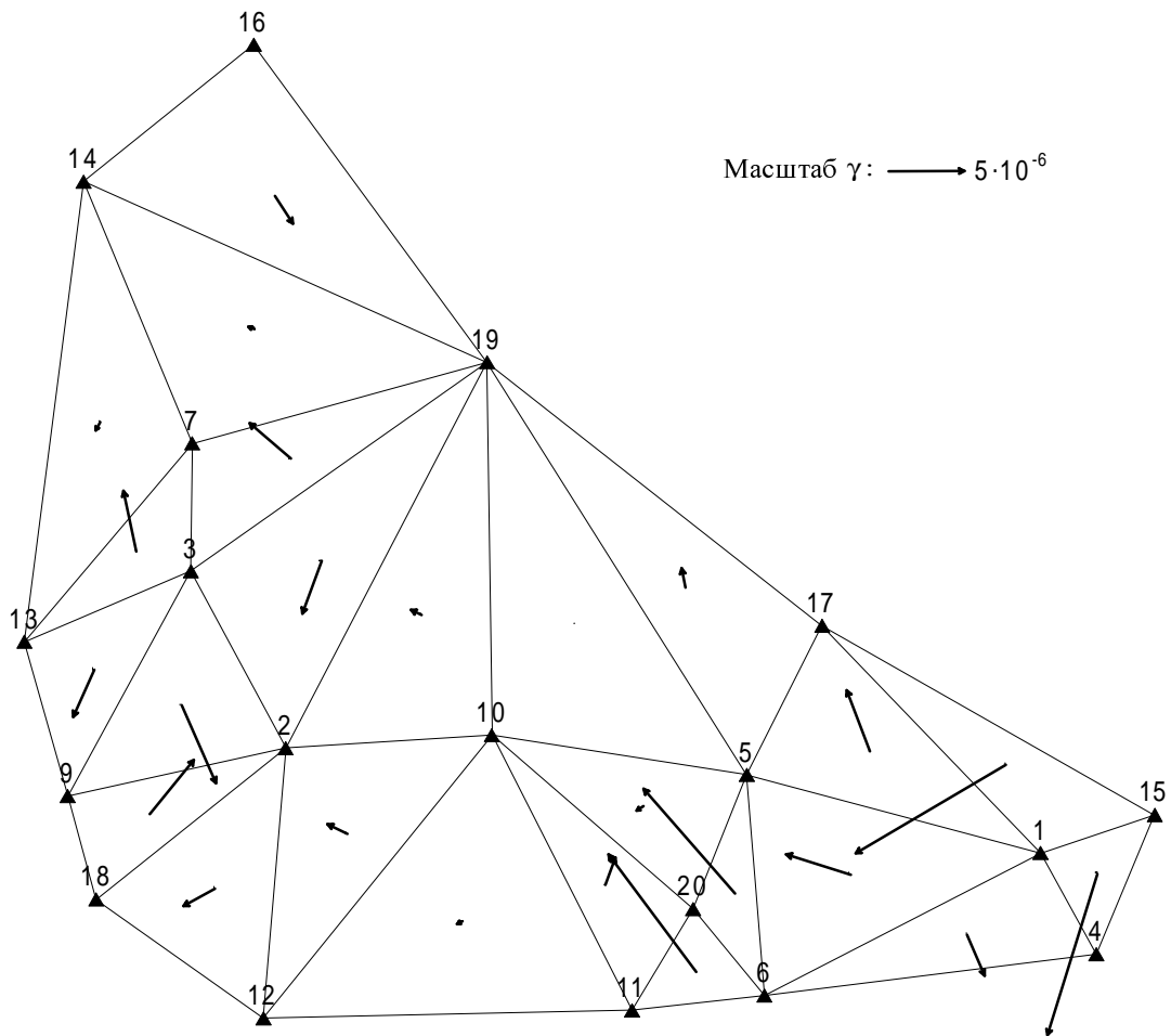
Рис.4. Розподіл відносного зсуву за результатами вимірювань циклів спостережень 1 – 4
