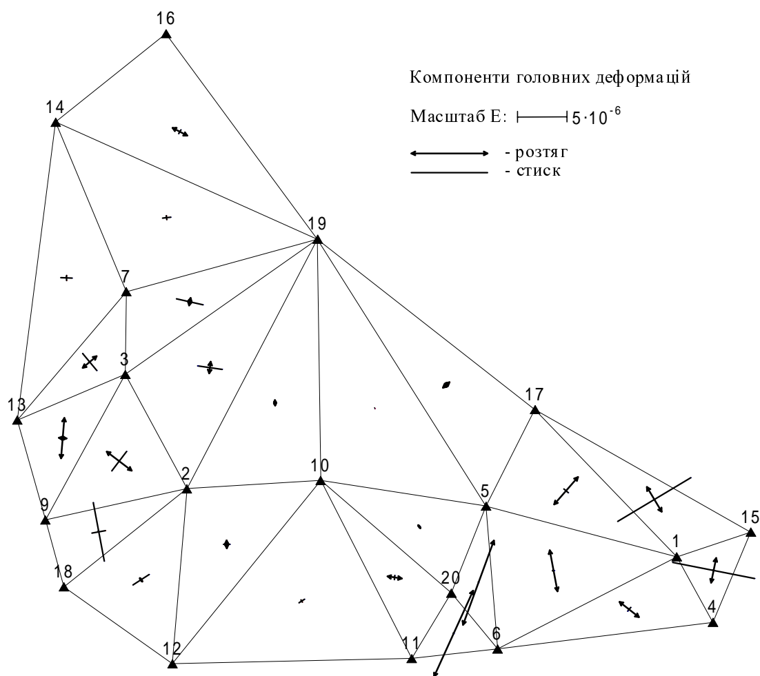
Рис.5. Розподіл екстремальних осей розтягу і стиску за результатами вимірів циклів спостережень 1 – 4
