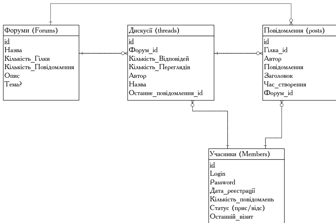
Рис. 1. Структура даних СУІН Веб-спільноти
