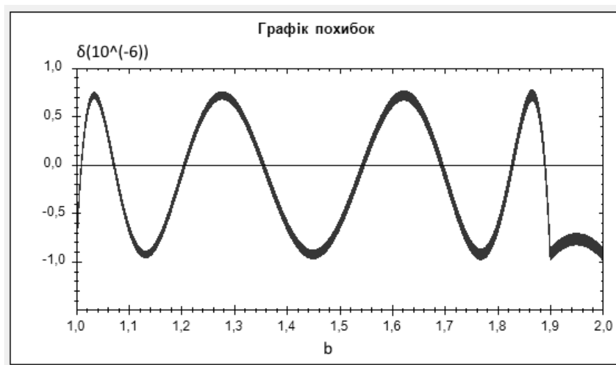
Рис. 1. Графік відносної похибки алгоритму 1 для a=1, b \in [1,2)
