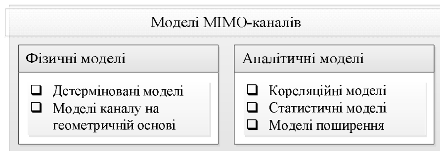
Рис. 2. Математичні моделі MIMO-каналу
