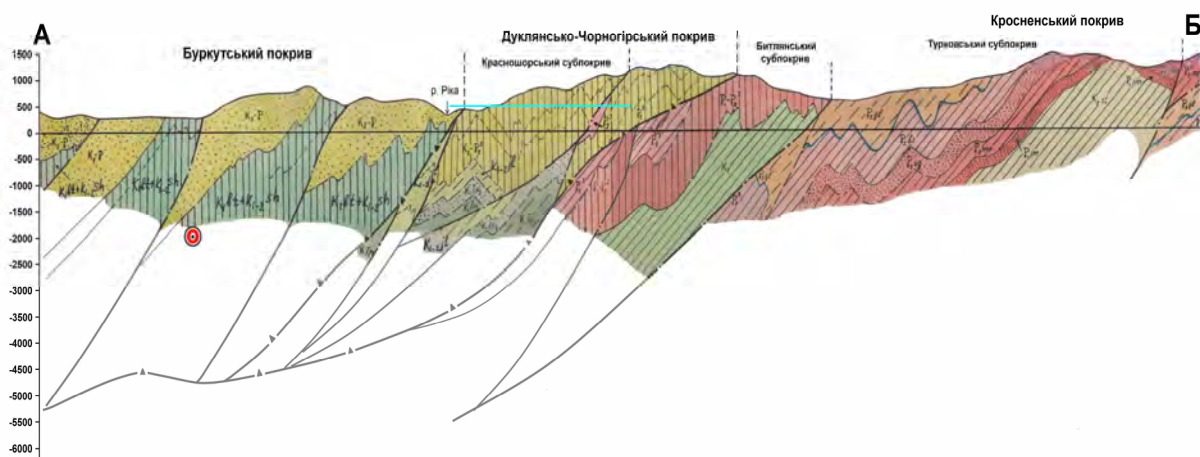
Рис. 3. Геологічний розріз по профілю Нижній Бистрий – Колочава (район Теребле-Ріцької ГЕС) Склали: В. Кузовенко, В. Шлапінський. Тут: — — проекція на розріз Вільшанського водосховища на ріці Тереблї; ● — вогнище неглибокого землетрусу в зоні профілю (інші пояснення в тексті).
