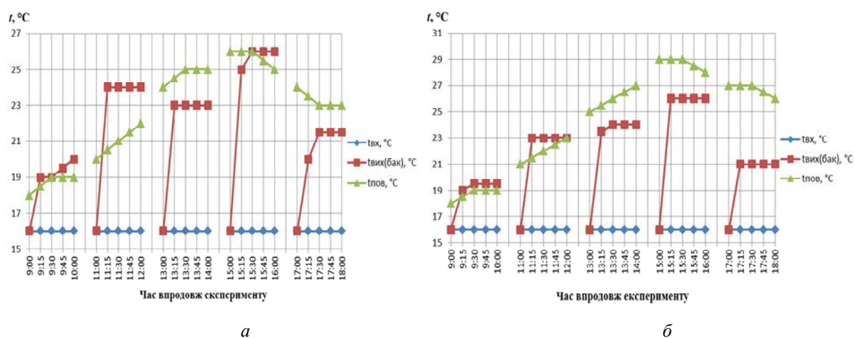
Рис. 2. Зміна температури теплоносія та температури зовнішнього середовища впродовж експерименту південно-західна (а) та південно-східна (б) орієнтація
