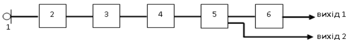
Рис. 5. Структурна схема пристрою для вимірювання параметрів акустичної емісії: 1 – н'єзоперетворювач; 2 – попередній підсилювач; 3 – блок фільтрів; 4 – основний підсилювач; 5 – дискримінаатор; 6 – детектор
