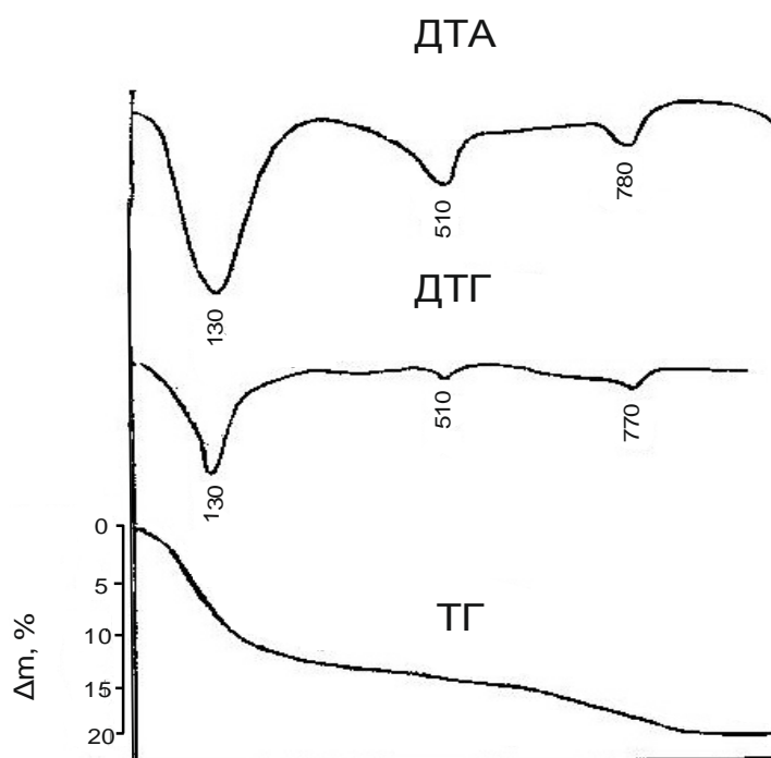
Рис. 2. Дериwатограма цеолітвмісного композиційного цементу, гідратованого 28 діб
