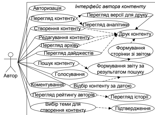
Рис. 7. Діаграма варіантів використання для інтерфейсу авторів контенту до інформаційного ресурсу в системах електронної контент-комерції
