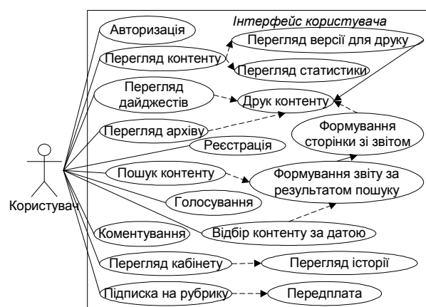
Рис. 5. Діаграма варіантів використання для інтерфейсу з обмеженим доступом користувача до інформаційного ресурсу в системах електронної контент-комерції
