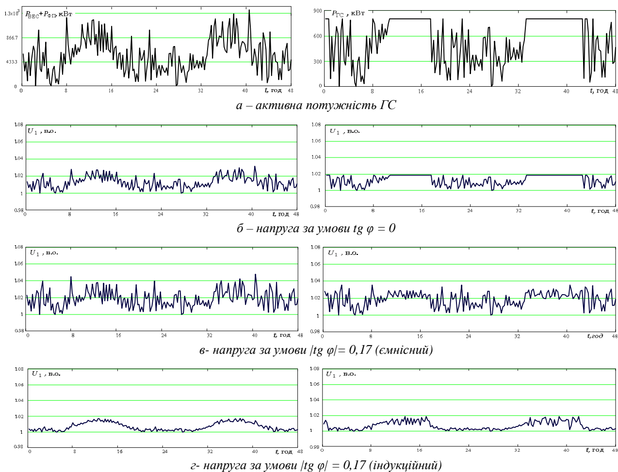
Рис. 5. Зміни напруги в пункті спільного приєднання за умови роботи вітрового та фотоелектричного генераторів
