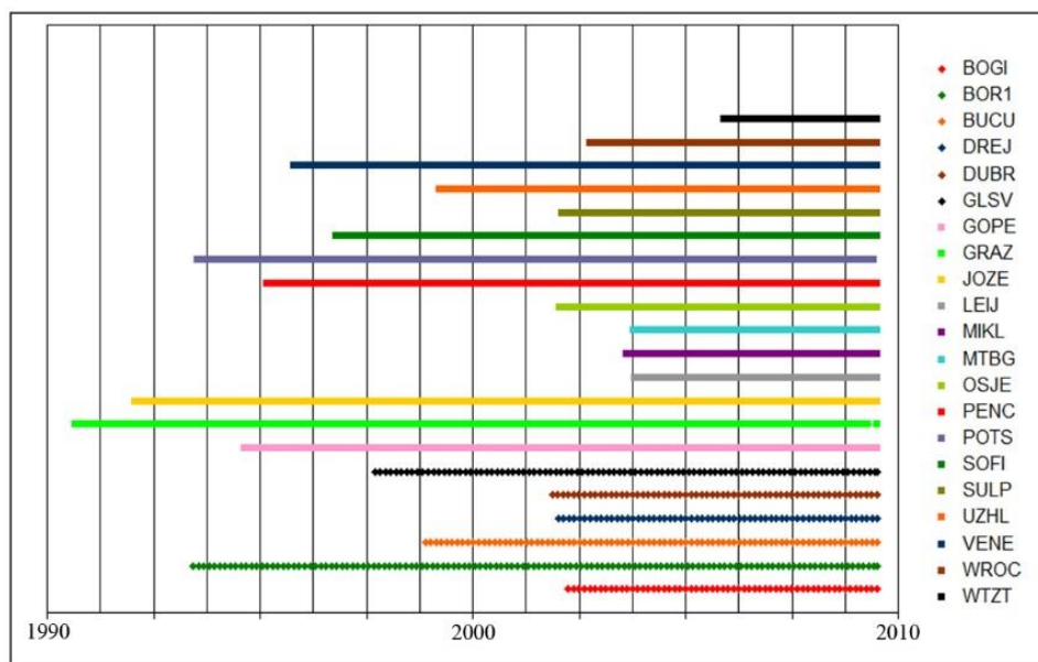
Рис. 2.16 Тривалість роботи перманентних ГНСС станцій, розташованих в регіоні Карпато-Балканської дуги
