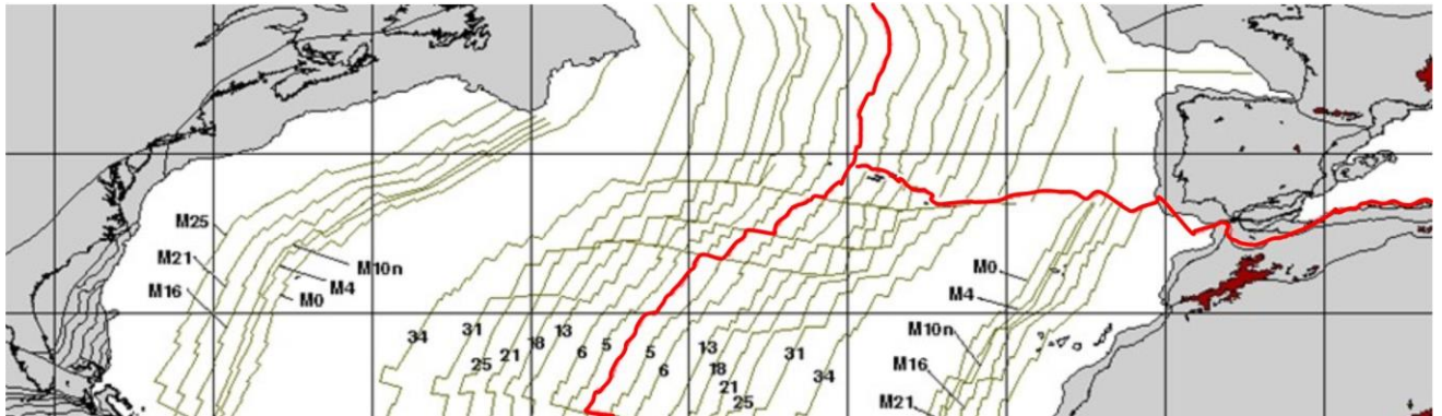
Рис. 3.23 Ізохрони для Центральної Атлантики. Лінії вказують на відносну позицію Північно-Американської плити відносно до Європейської [88]
