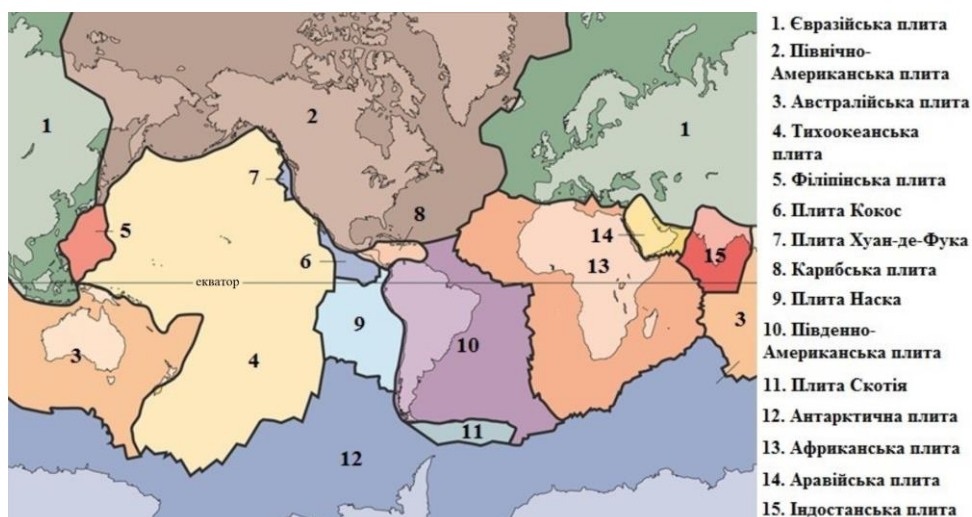
Рис. 1.2 Схема розташування основних літосферних плит [110]
