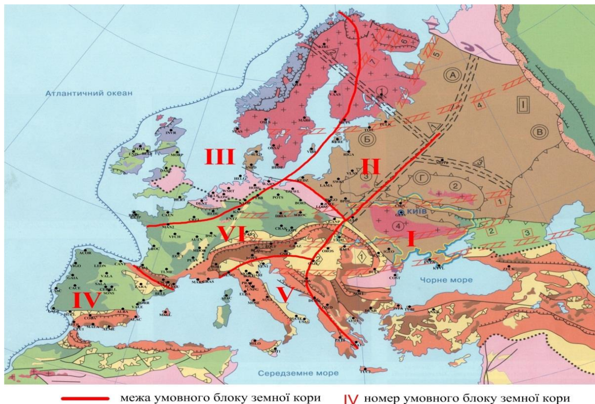
Рис. 2.13 Схема поділу території Європи на умовні блоки земної кори
