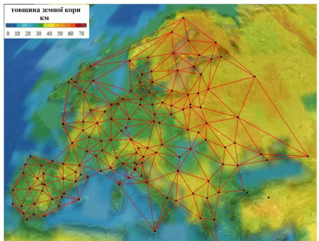
Рис. 2.22 Мережі трикутників перманентних ГНСС-станцій на території Європи за період з 2001 по 2010 роки
