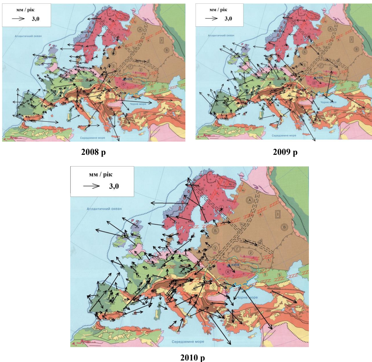
Рис. 2.12 Карти-схеми розподілу щорічних векторів РШГР перманентних ГНСС-станцій на території Європи за період з 2000 по 2010 рік
