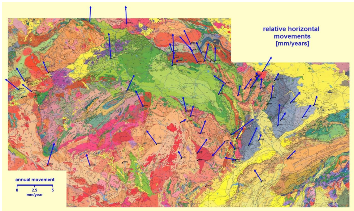
Рис. 2.1 Карта річних горизонтальних рухів Богемського масиву [86]
