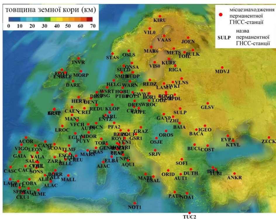
Рис. 2.8 Схема розташування постійних ГНСС-станцій Європи, використаних у дослідженні
