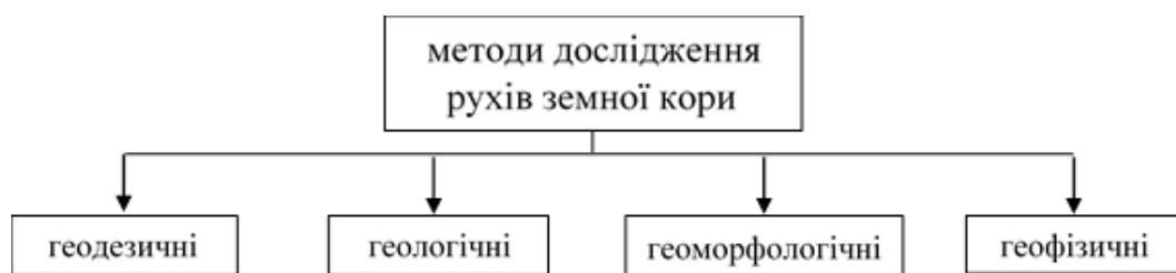
Рис. 1.6 Основні методи вивчення рухів земної кори
