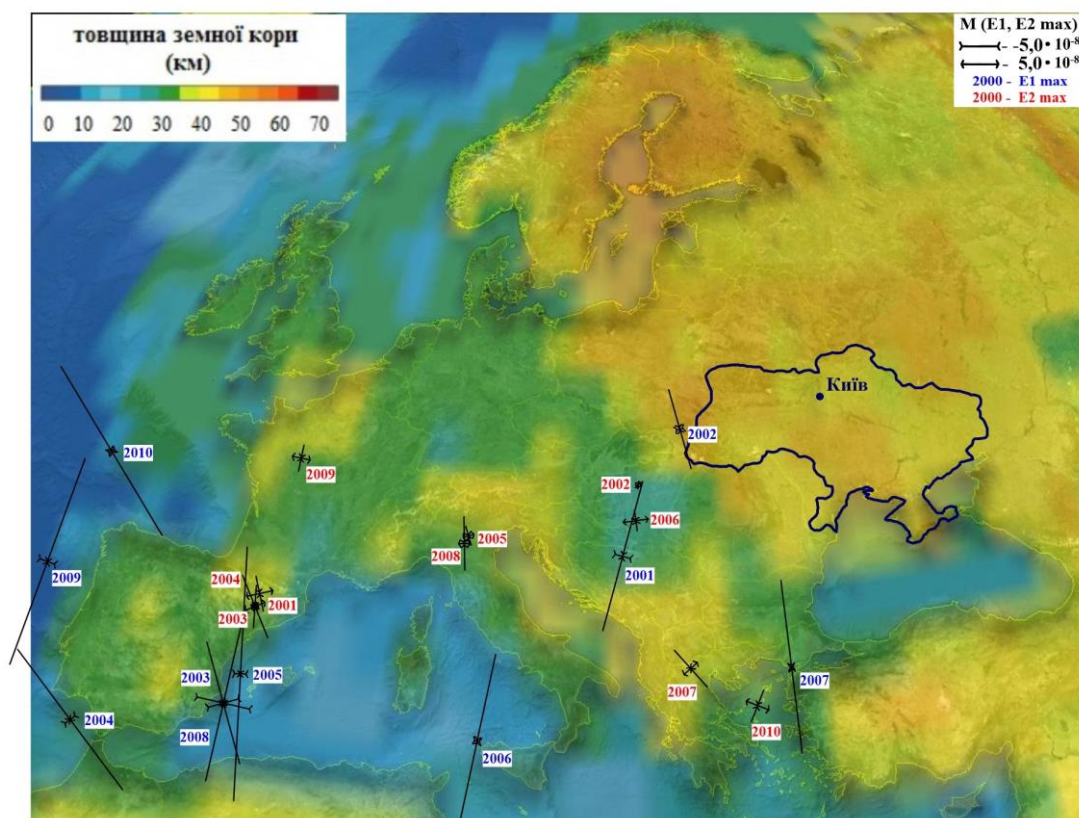
Рис. 2.28 Карта-схема розподілу максимальних значень E_1 та E_2 ( 10^{-8}/\text{рік} ) на території Європи за період з 2000 по 2010 роки
