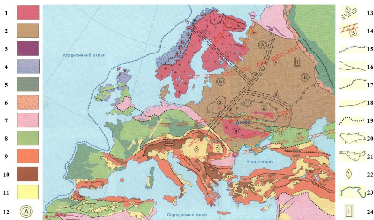
Рис. 1.4 Фрагмент тектонічної карти для території Європи
