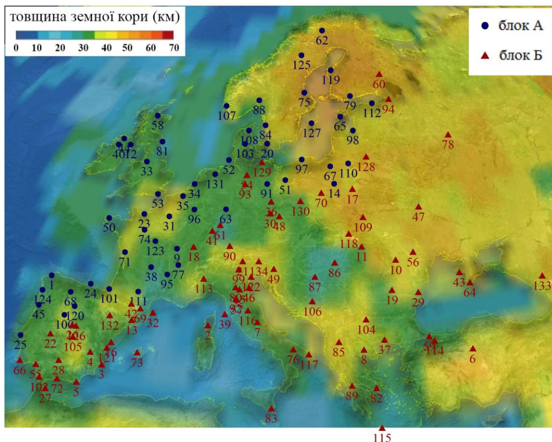
Рис. 3.19 Просторовий розподіл ГНСС-станцій блоків А та Б
