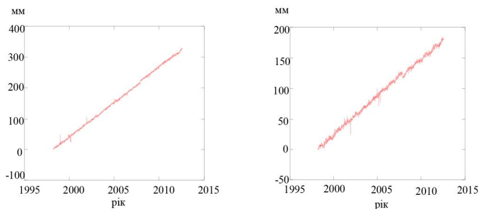
Рис. 2.9 Часовий ряд постійної ГНСС-станції GLSV (зміна значення V_B та V_L за період з 1998 по 2012 роки)
