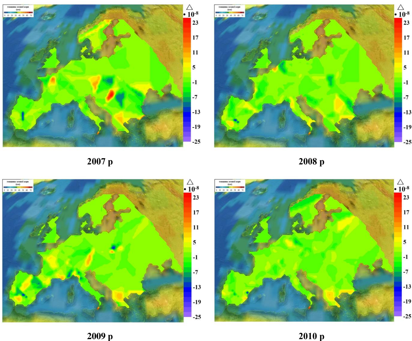
Рис. 2.25 Карти-схеми щорічного розподілу дилатації земної кори території Європи за період з 2001 по 2010 роки
