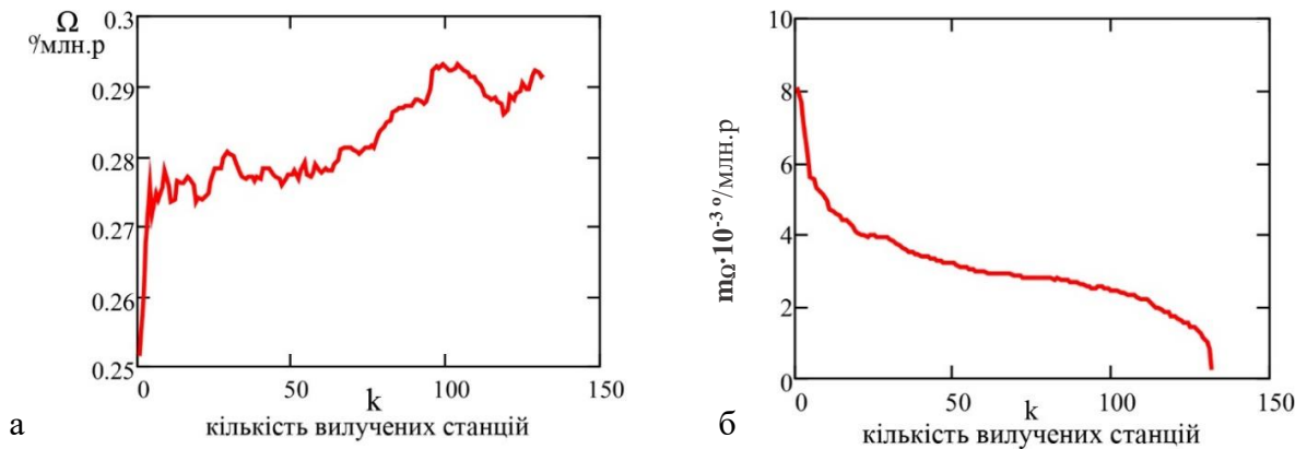
Рис. 3.3 Зміна кутової швидкості \Omega обертання плити (а) та її m_\Omega (б) від кількості вилучених з сукупності станцій
