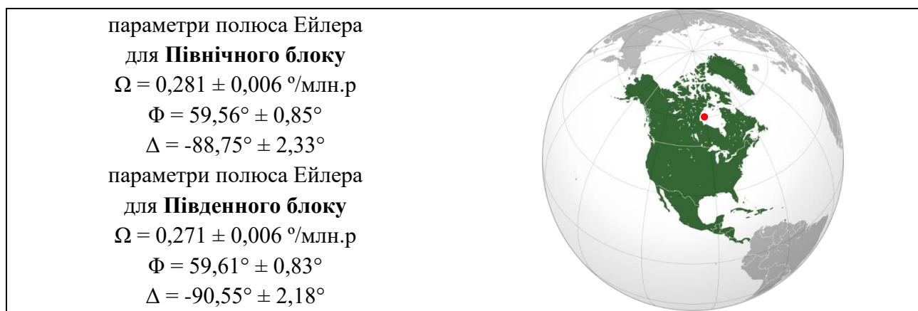
Рис. 3.20 Параметри та місцезнаходження полюса Ейлера для Північного та Південного блоків
