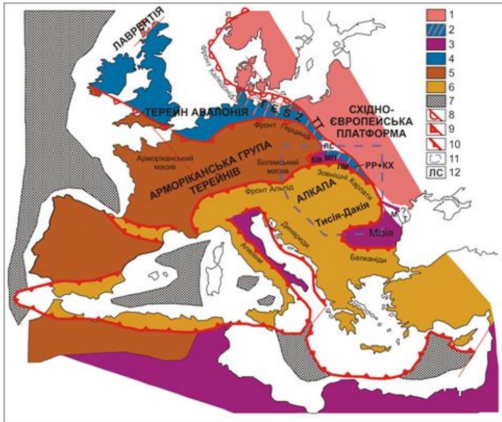
Рис. 3.25 Структурний поділ Європи. Складено за матеріалами [195, 19, 34, 107, 71, 121, 96, 1, 10] та ін.
