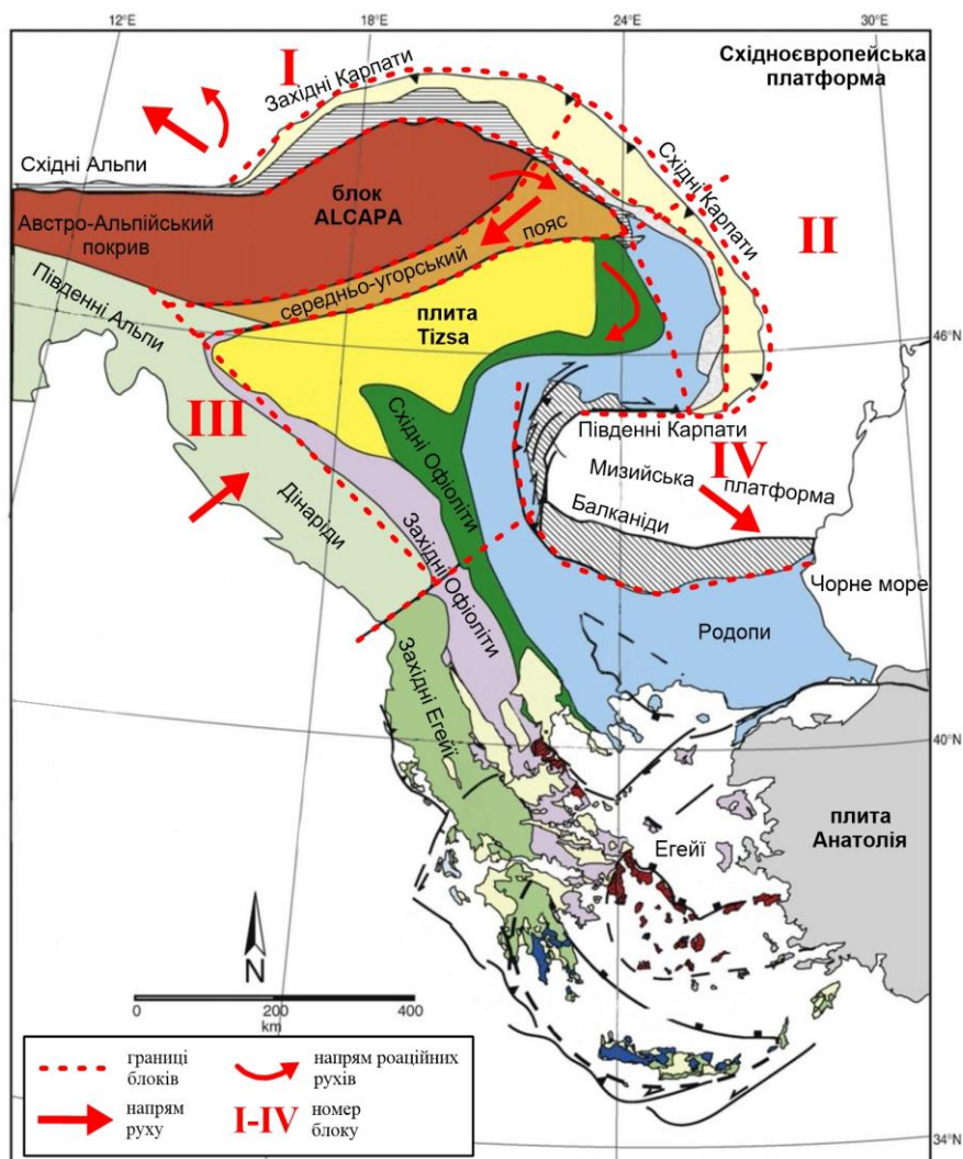
Рис. 2.20 Геодинамічна схема сучасної тектонічної активності земної кори у Карпато-Балканському регіоні та прилеглих територіях
