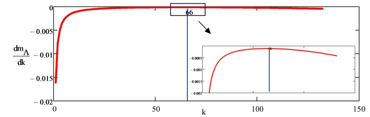
Рис. 3.15 Функція похідної \frac{dm_{\Delta}}{dk}
