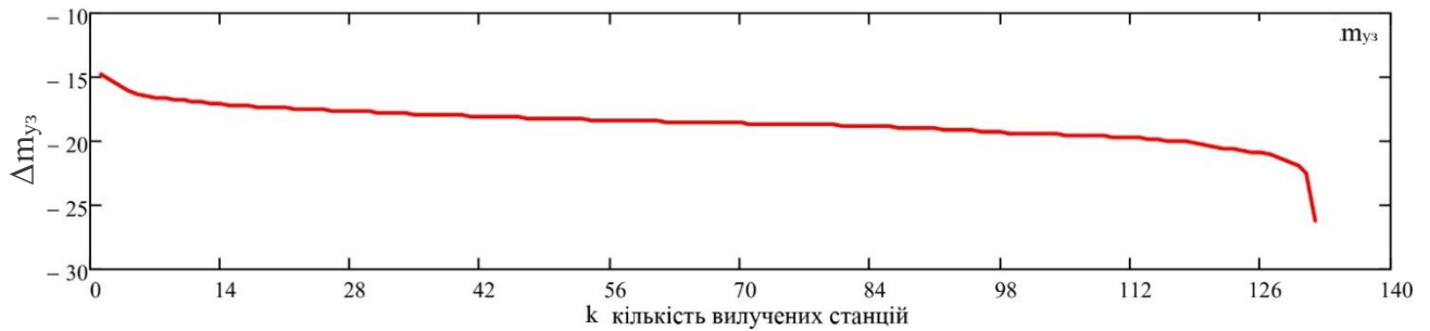
Рис. 3.6 Зміна узагальненого параметру \Delta m_{уз} від кількості вилучених з сукупності станцій
