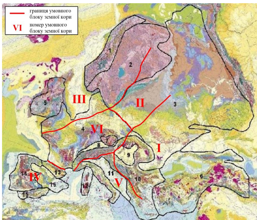
Рис. 2.14 Диференціація території Європи на УБЗК та деференціація за Vednarek'ом на основі результатів ГНСС-спостережень
