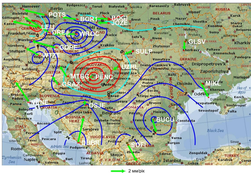
Рис. 2.19 Залишкові просторові рухи перманентних ГНСС-станцій після зняття регіонального трендового впливу
