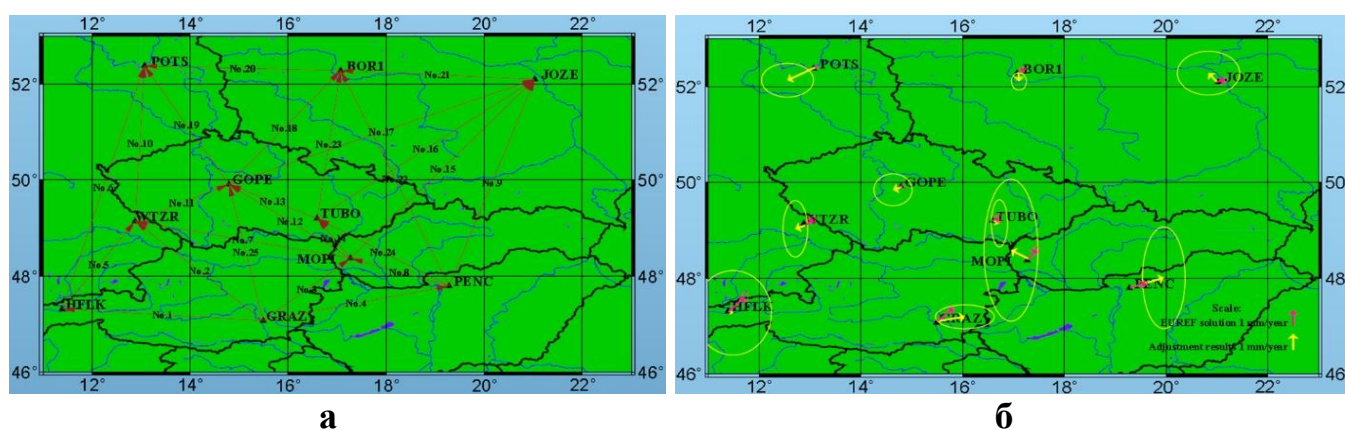
Рис. 2.3 Мережа дослідження та річні горизонтальні швидкості ГНСС станцій [74]
