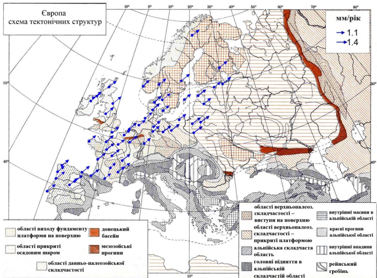
Рис. 3.22 Схема модельних векторів швидкостей ГРЗК Північного блоку відносно Південного (нерухомого)
