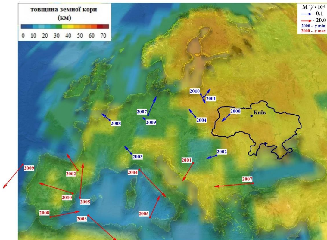
Рис. 2.27 Карта-схема розподілу мінімальних та максимальних значень загального зсуву земної кори ( \gamma \times 10^{-8}/\text{рік} ) на території Європи за період 2000 – 2010 роки
