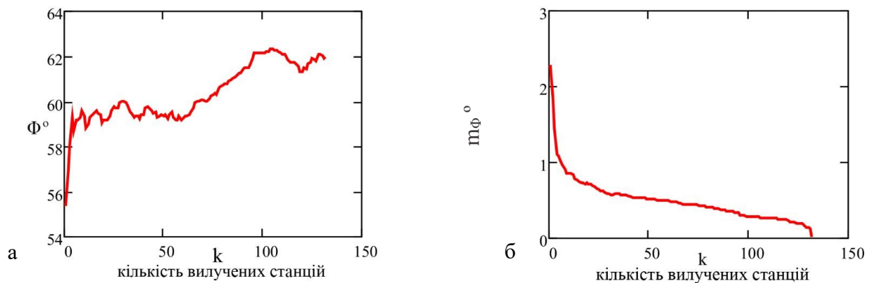
Рис. 3.4 Зміна широти \Phi полюса Ейлера (а) та її m_\Phi (б) від кількості вилучених з сукупності станцій
