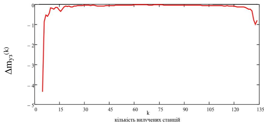
Рис. 3.7 Зміна градієнтів функції \Delta m_{уз}^{(k)}
