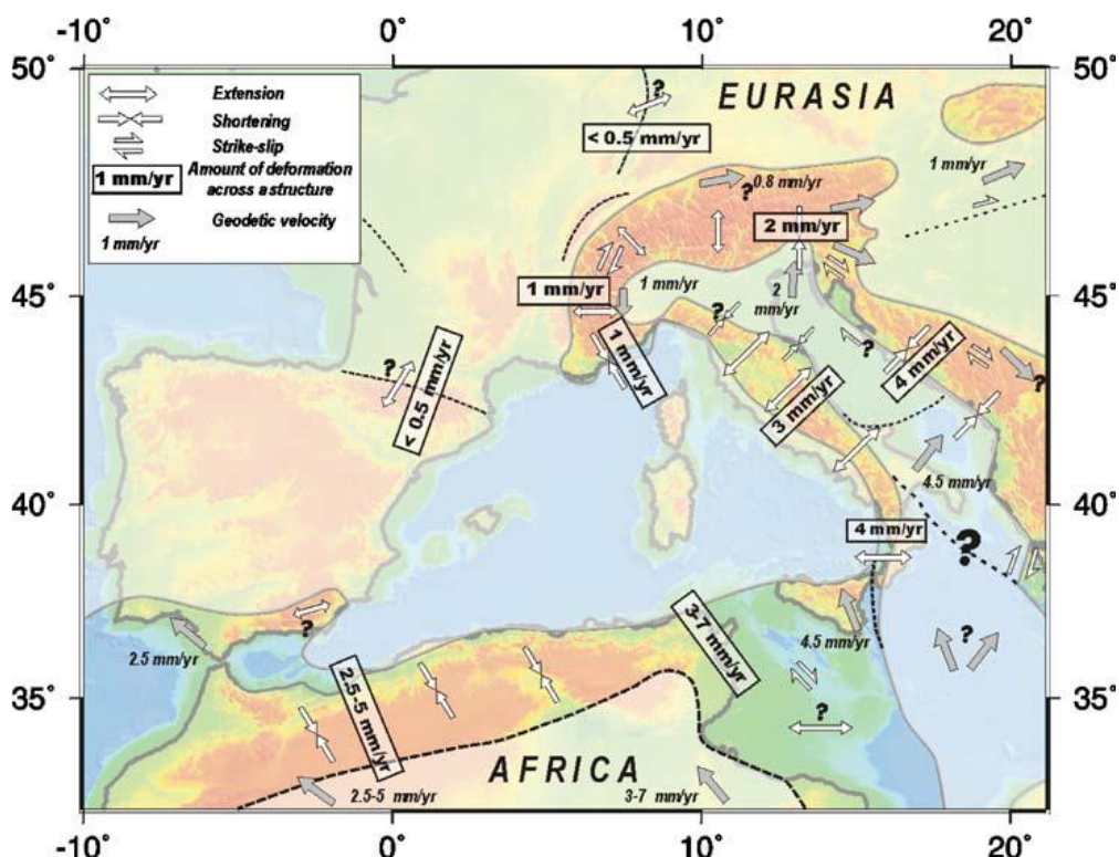
Рис. 2.6 Виділені зони та їх швидкості деформації на території Європи та західного середземномор'я [73]
