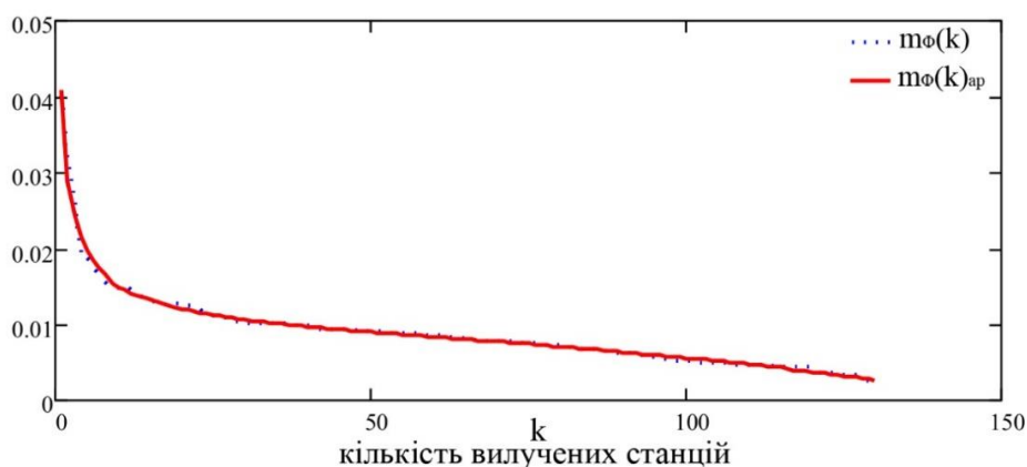
Рис. 3.11 Функція m_{\Phi}(k) та функція m_{\Phi}(k)_{\text{ап}}
