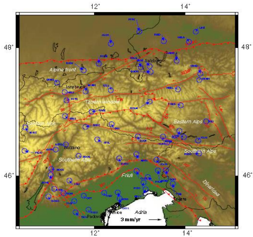
Рис. 2.2 Швидкості горизонтальних рухів Альпійського поясу [69]
