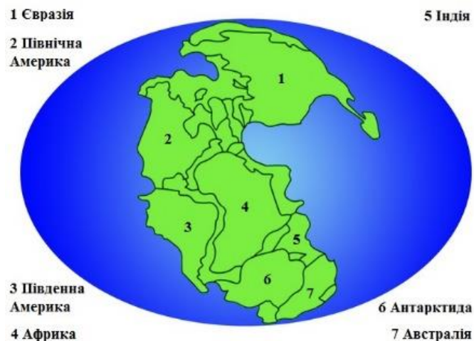
Рис. 1.1 Суперконтинент Пангея. Розташування сучасних континентів 200 мільйонів років тому
