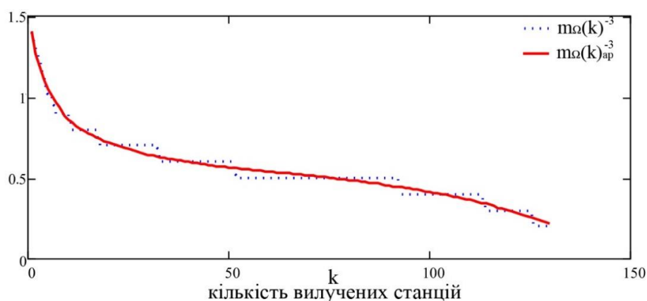
Рис. 3.10 Функція m_{\Omega}(k) та функція m_{\Omega}(k)_{\text{ап}}
