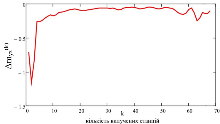
Рис. 3.17 Зміна градієнтів функції \Delta m_{уз}(k) для сукупності Б
