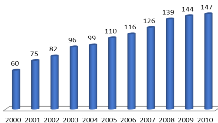
Рис. 2.7 Щорічна кількість перманентних ГНСС-станцій, використаних у дослідженні
