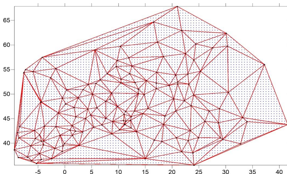
Рис. 2.24 Схема мережі трикутників перманентних ГНСС-станцій з точками, в яких обчислено параметри горизонтальної деформації земної кори (• – точки, для яких обчислені параметри деформації земної кори)
