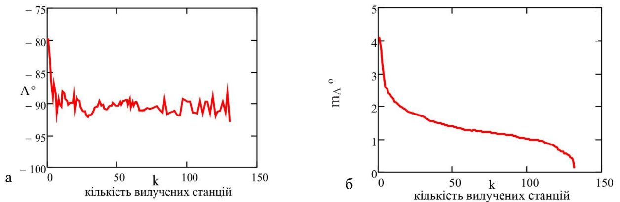
Рис. 3.5 Зміна довготи \Lambda полюса Ейлера (а) та її m_\Lambda (б) від кількості вилучених з сукупності станцій
