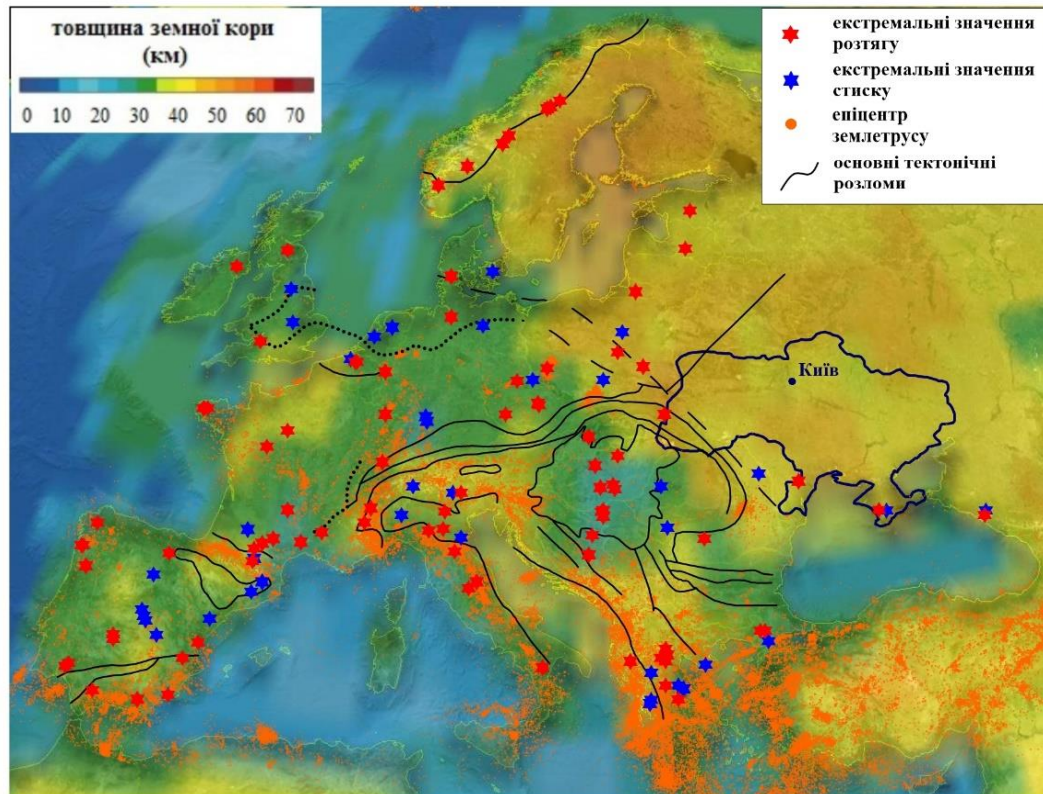
Рис. 2.26 Карта-схема розподілу екстремальних значень швидкостей дилатації земної кори 10^{-8}/\text{рік} та прояву сейсмічної активності на території Європи за період з 2000 по 2010 роки
