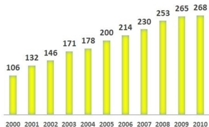
Рис. 2.23 Річна кількість трикутників у мережі трикутників перманентних ГНСС-станцій, використаних у дослідженні
