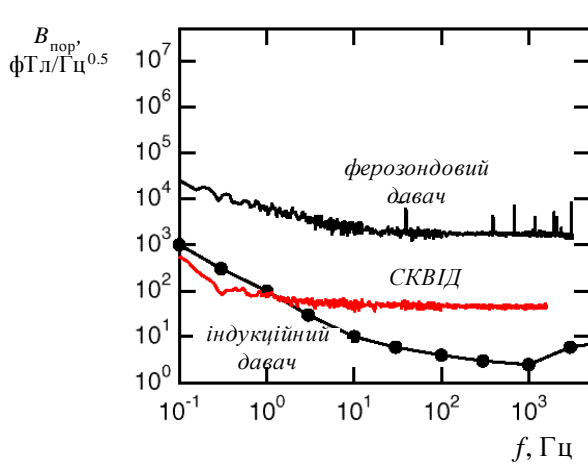
Рис. 2. Рівень густини еквівалентного шумового поля для трьох давачів під час вимірювань в екрані
