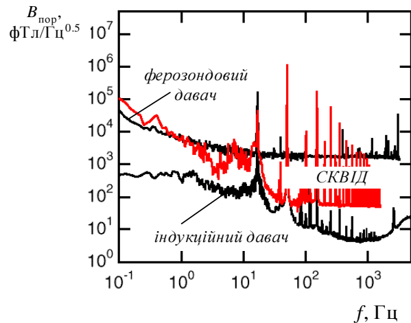
Рис. 3. Рівень густини еквівалентного шумового поля для трьох давачів під час вимірювань у сільській місцевості без екрана
