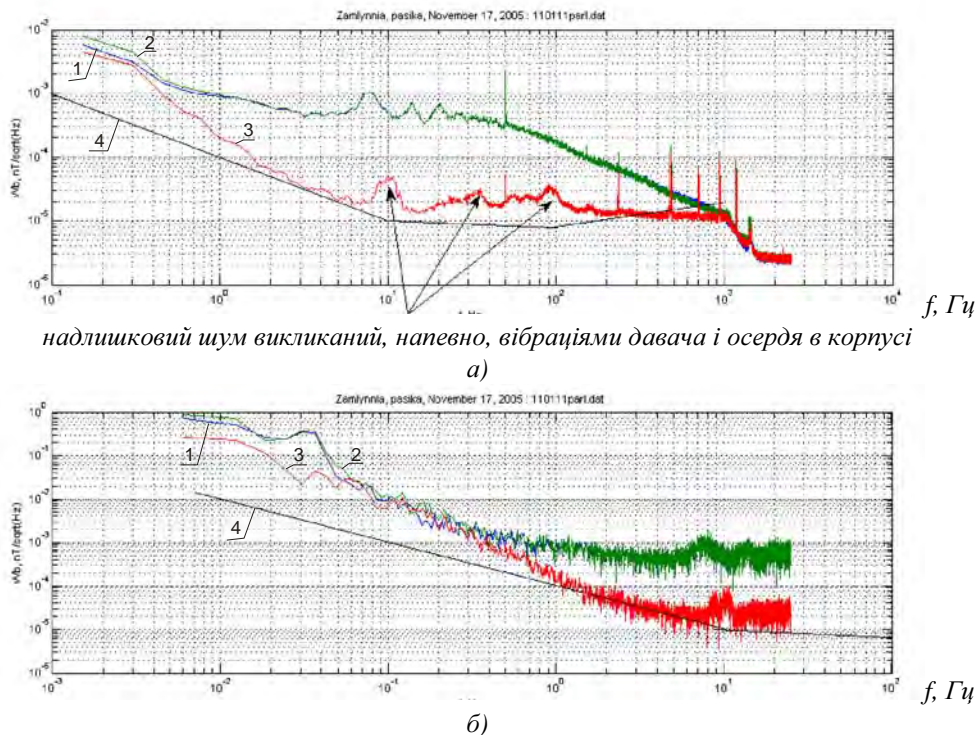
Рис. 11. Результати вимірювань: а – в частотному діапазоні 10^{-1} - 10^3 Гц; б – в частотному діапазоні 10^{-2} - 10^2 Гц
