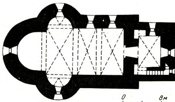
Рис. 34. Церква св. Онуфрія в урочищі (план)
