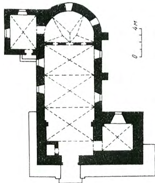
Рис. 31. Успенська церква в Уневі (план)
