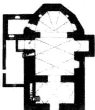
Рис. 1. План П'ятницької церкви
