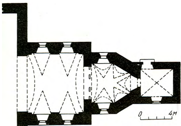
Рис. 17. Церква св. Миколая в Теробовлі (план)
