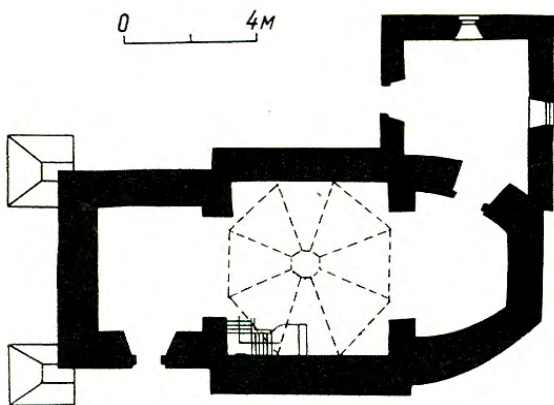
Рис. 15. Успенська церква с. Кошилівці (план)
