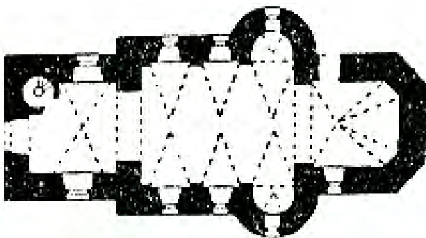
Рис. 25. Миколаївська церква в Бучачі (план)
