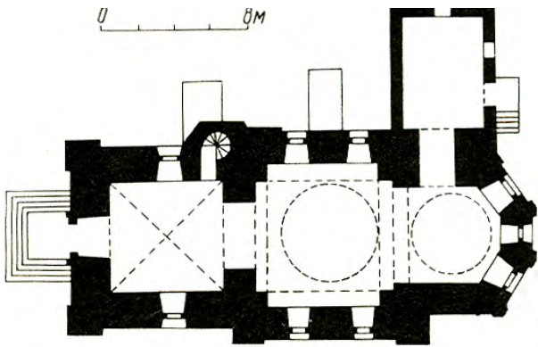
Рис. 20. Успенська церква в Підгайцях (план)
