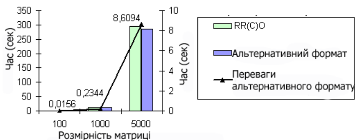
Рис. 2. Залежність витрат часу на пакування матриці від розмірності матриці
