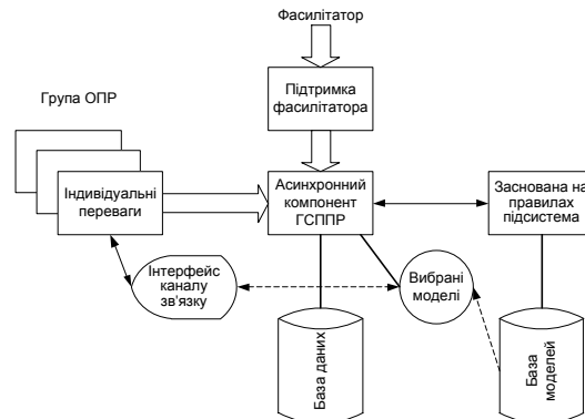
Рис.1. Архітектура ГСППР
