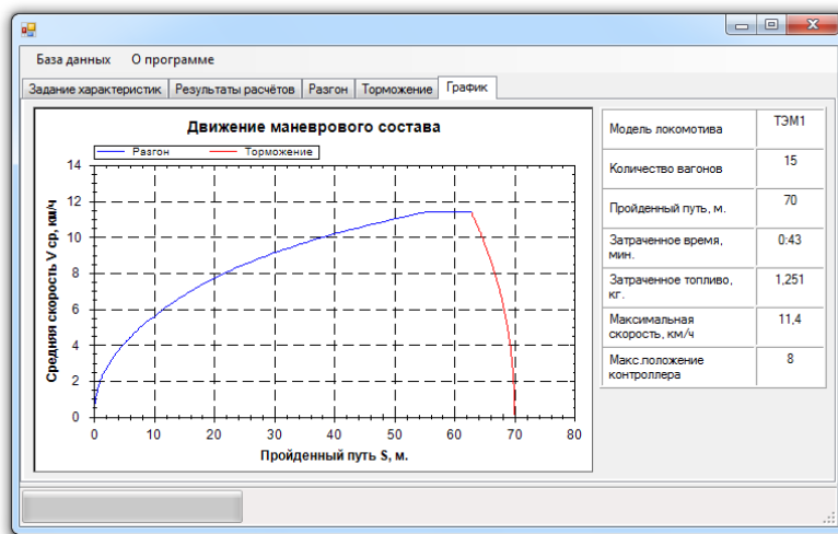
Рис.6. Окно «График»
