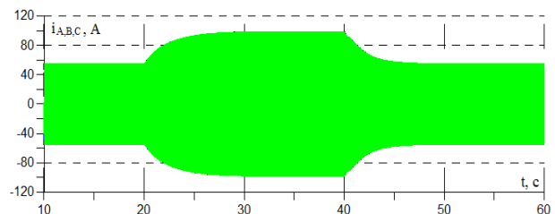
Рис. 8. Струм статора АД (миттєві значення)
