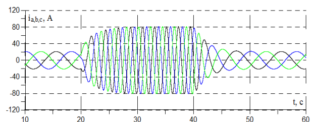
Рис. 9. Приведені до статора струми ротора (миттєві, значення)
