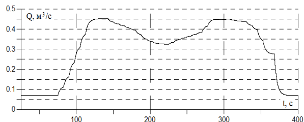
Рис. 12. Розрахункова витрата
