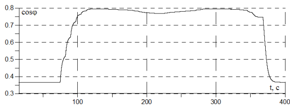
Рис. 16. Коефіцієнт потужності електроприводу
