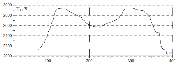
Рис. 18. Фазна напруга статора АД (діюче значення)
