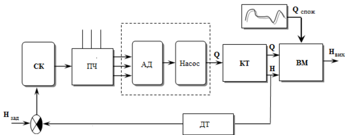
Рис. 1. Структурна схема системи керування:
