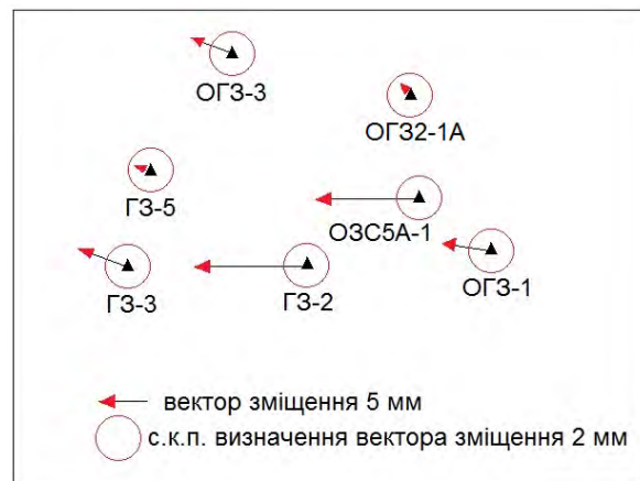
Рис. 2. Схема векторів горизонтальних зміщень пунктів каркасної геодезичної мережі Дністровської ГАЕС за період 2005–2014 рр.
