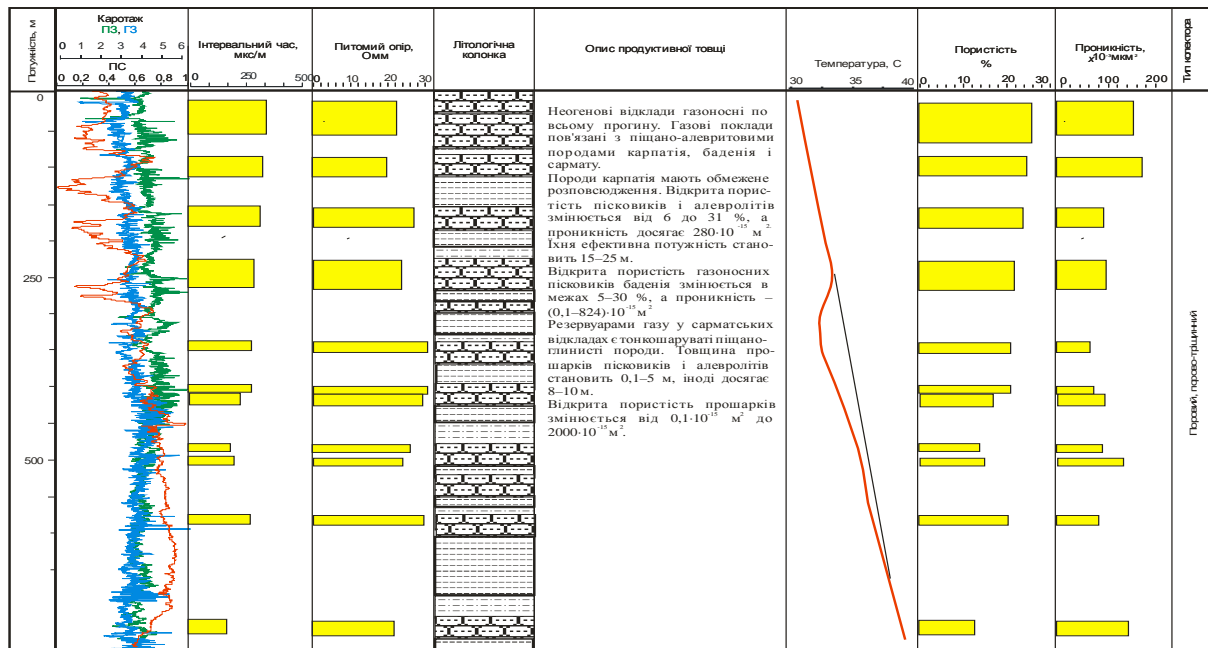
Рис. 1. Типовий геолого-петрофізичний розріз неогенових відкладів Зовнішньої зони Передкарпатського прогину
