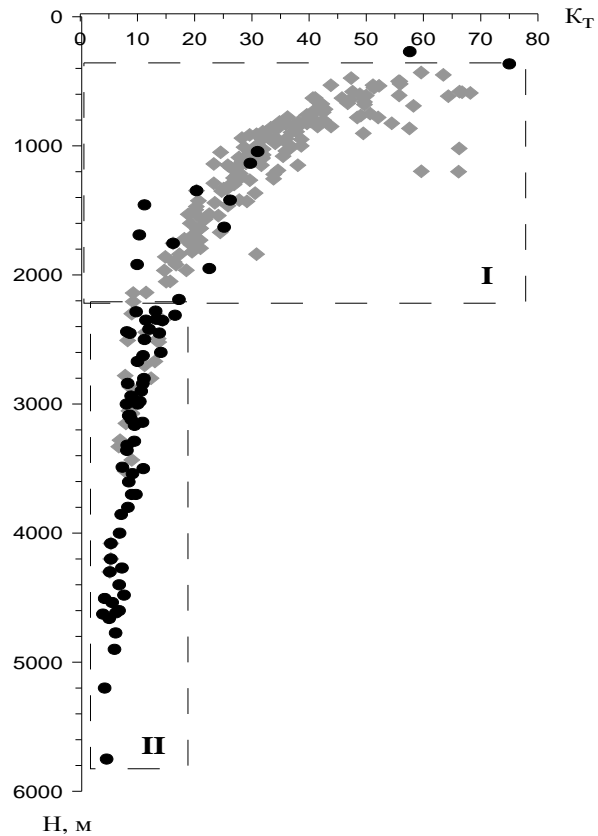
Рис. 2. Розподіл покладів вуглеводнів Західного регіону в залежно від термобаричного коефіцієнта ( K_m = T_{nT} / P_{nT} ) Поклади: ● – нафтові, ◆ – газові
