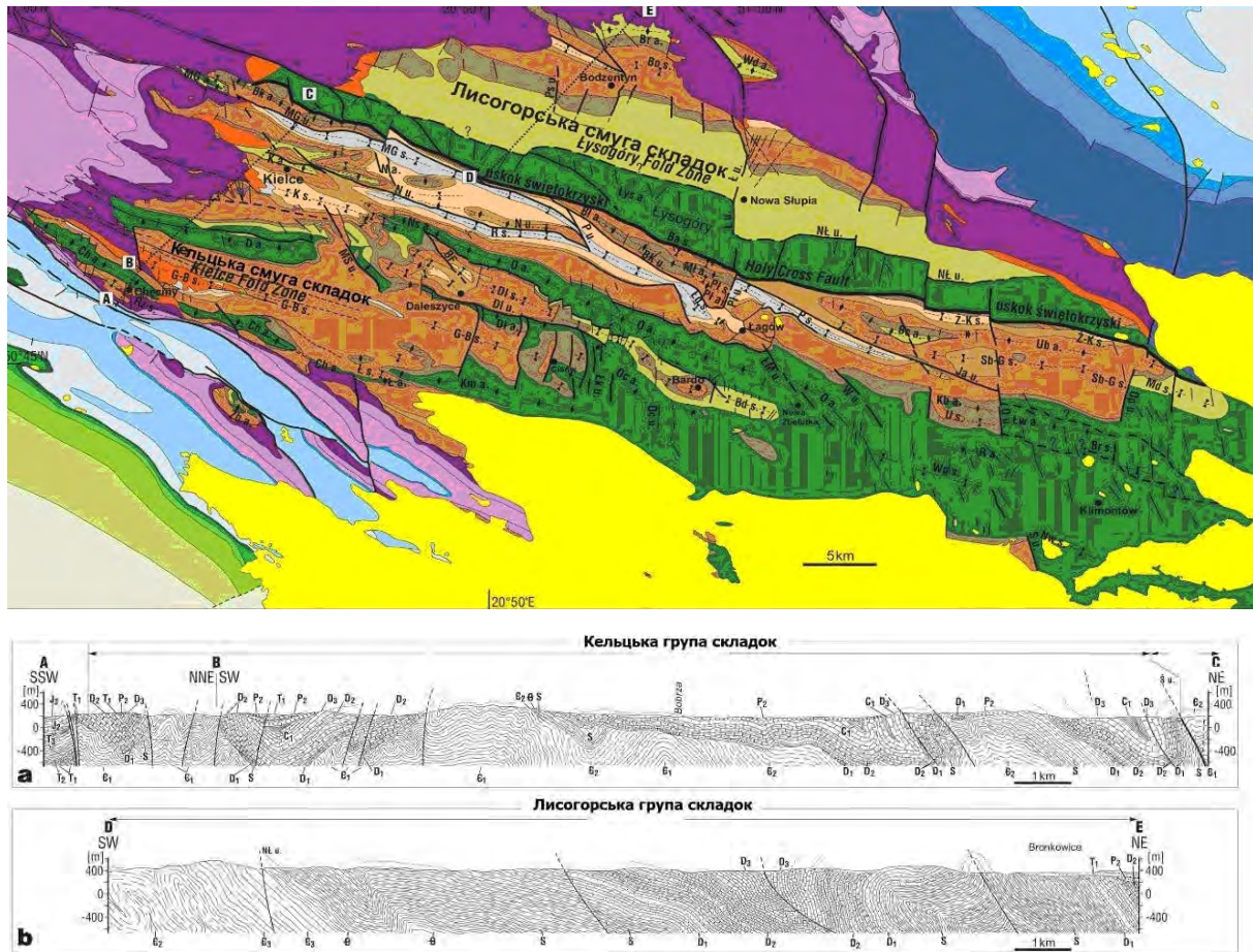
Рис. 2. Геологічна карта і профіль через кельцьку і лисогорську групи складок Свентокшицьких гір (А. Конон, 2008)
