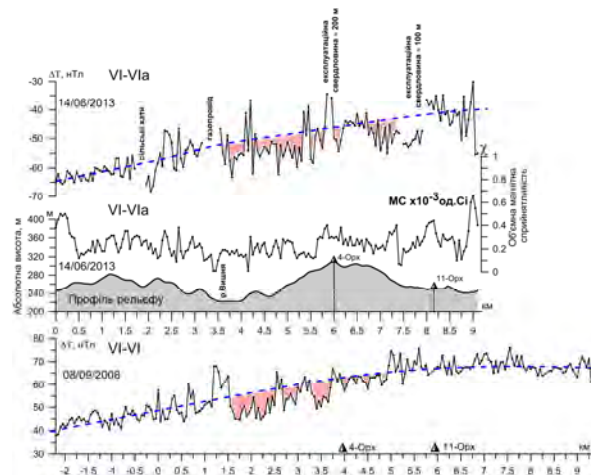
Рис. 2. Аномальне магнітне поле \Delta T_a ділянки локальних аномалій \Delta T_a (виділено червоним кольором), об’ємна магнітна сприйнятливості, профіль рельєфу на Орховицькій структурі.
