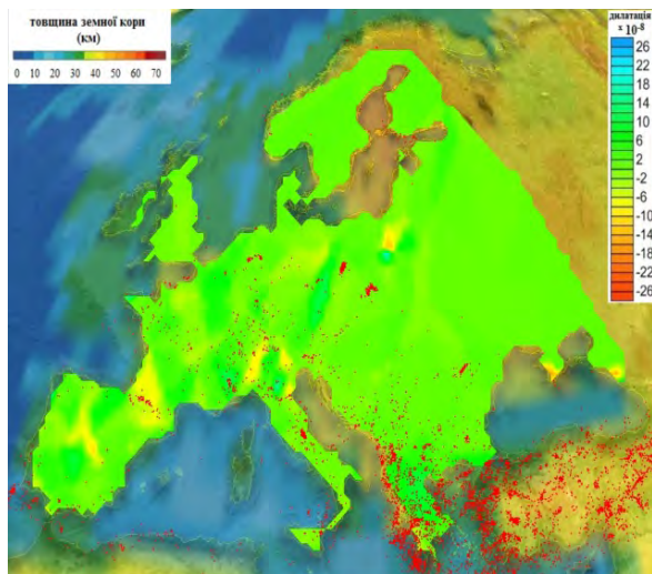
Рис. 4. Приклад карти-схеми розподілу швидкостей дилатації ( 10^{-8} /рік) та епіцентрів землетрусів на території Європи у 2009 році (• – епіцентри землетрусів)
