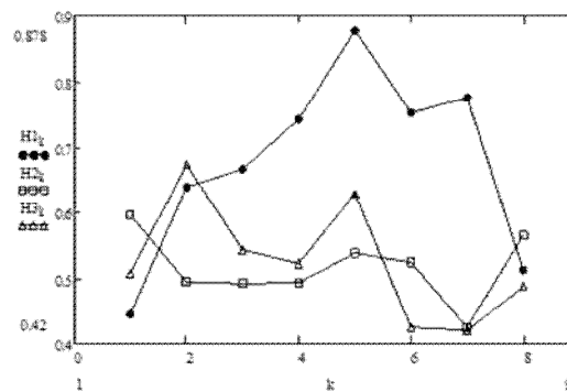
Рис. 6. Портрети Хьорста для трьох файлів із записаним шумом. Графіки з білими квадратами і трикутниками відповідають аудіоплаті стаціонарного комп'ютера, графік з чорними точками відповідає аудіоплаті нетбука
