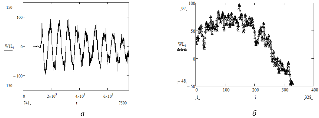
Рис. 3. Власні шуми мікрофона: а – амплітуда шумів мікрофону залежно від часу; б – ділянка графіка (а) в околі відліків t=2440
