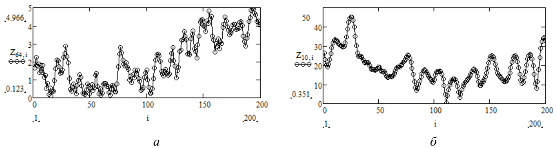
Рис.4. Динаміка змін спектральних компонент шуму: а – для 64-ї компоненти; б – для 10-ї компоненти
