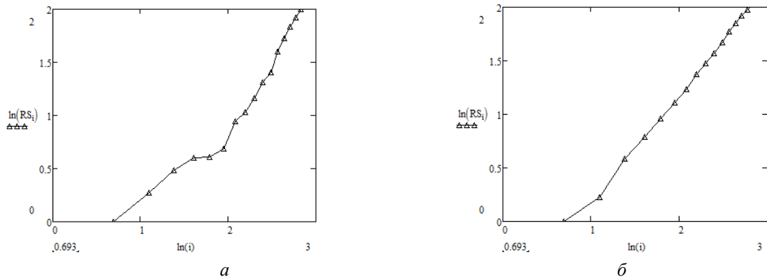
Рис.5. Графік RS статистики спектральних компонент шуму: а – для 64-ї компоненти; б – для 10-ї компоненти
