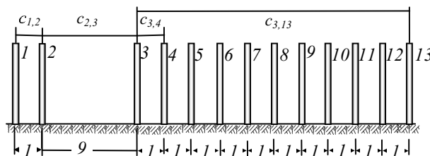
Рис. 4. Схема розташування трубчастих знаків базиса Біля верху труб їхні номери. Внизу інтервали подані в метрах
