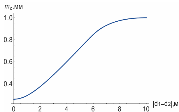
Рис. 3. Вплив нерівності плечей на точність визначення десятиметрового інтервалу базиса Fig. 3. The impact of shoulders inequality on the accuracy of 10 meter interval basis determine
