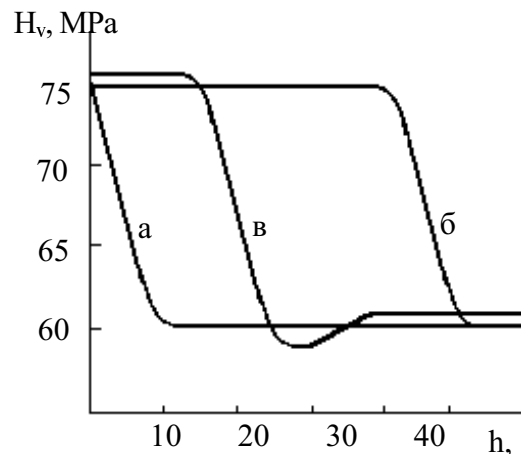
Рис. 8. Апроксимовані криві залежності мікротвердості від глибини в зразках CdTe. E , Дж/см 2 : а - 2,9; б - 3,2; в - 3,0.
