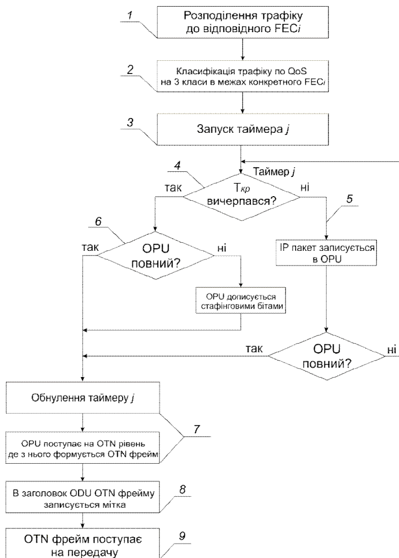
Рис. 4. Алгоритм агрегації вхідного трафіку від мереж доступу
