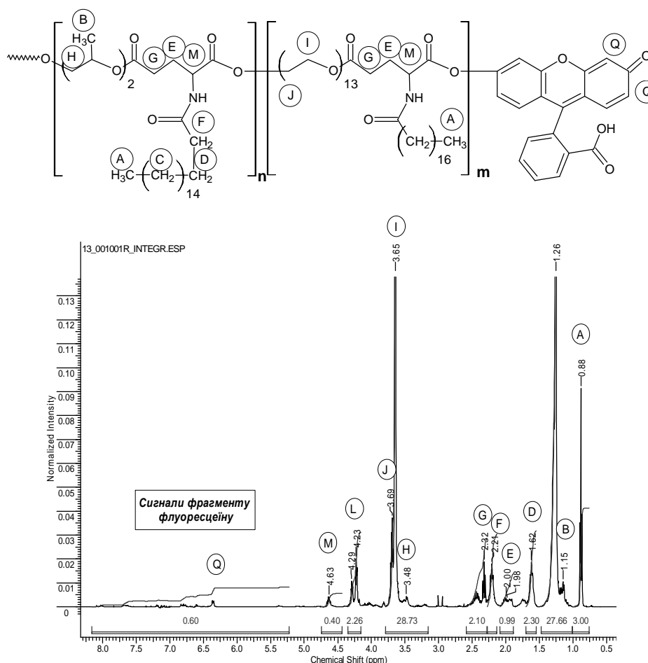
Рис. 2. ^1\text{H} ЯМР спектр кополієстеру co-GluSt-co-PEG-400-co-DPG-Fl (розчинник хлороформ, 300 МГц)
