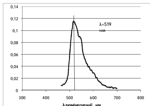
Рис. 3. Спектри люмінесценції а -водно-спиртового розчину та б -октанольного розчину кополіестеру з флуоресцентними фрагментами co-Glu(St)-co-PEG400-co-DPG-Fl .
