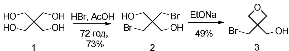
Рис. 2. Одержання вихідного 3-бромометил-3-гідроксиметил-оксетану
