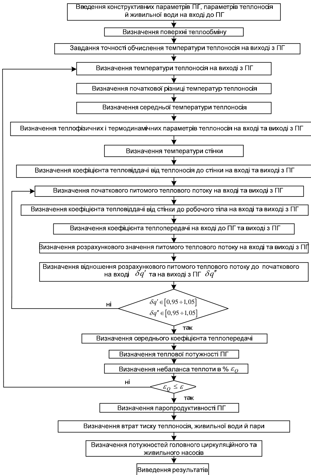
Логіко-структурна блок-схема математичної моделі горизонтального парогенератора
