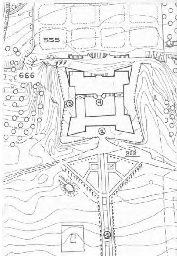
Рис. 1. Генеральний план
