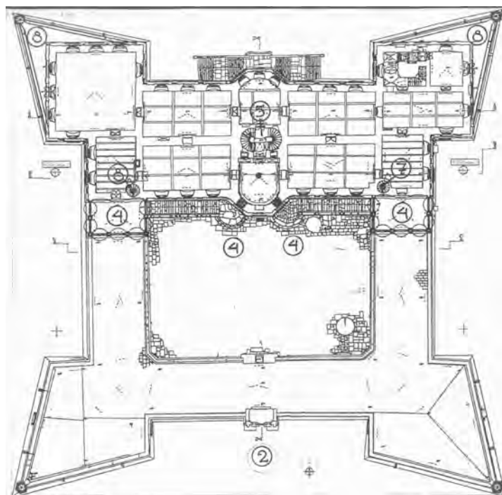
Рис. 4. План другого поверху
