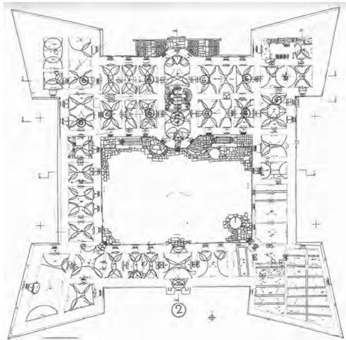
Рис. 3. План першого поверху
