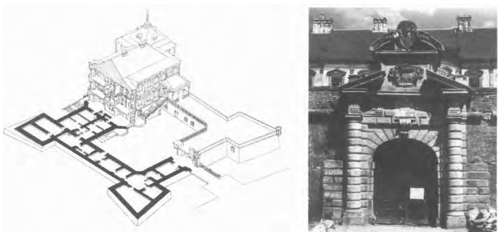
Рис. 2. Аксонометрія та в'їзна брама [1, с. 166]
