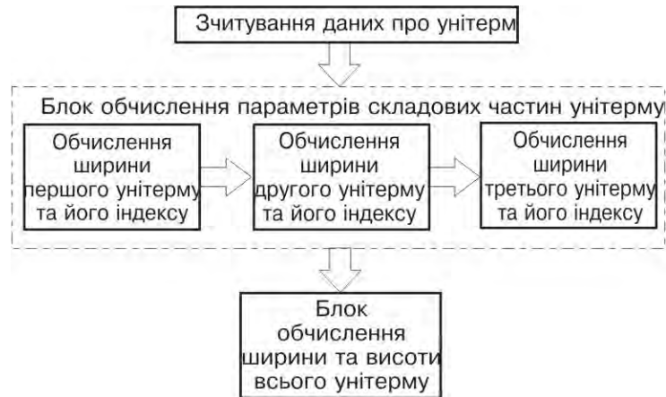
Рис. 1. Схеми алгоритму обчислення геометричних розмірів унітерму
