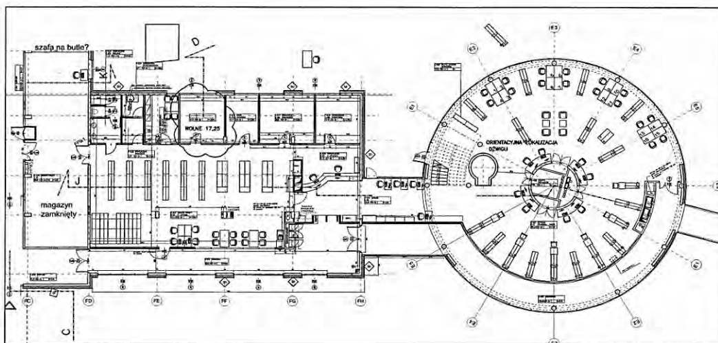
Rys. 1A. Plany pomieszczeń nowej biblioteki – parter.
