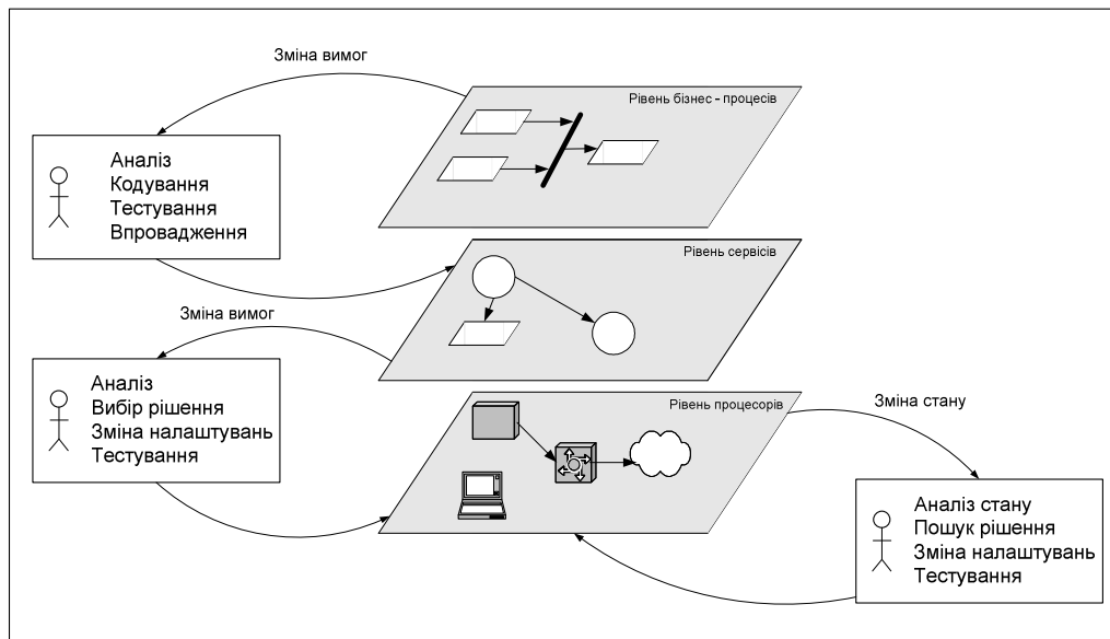
Рис. 1. Багаторівнева концептуальна модель програмної системи
