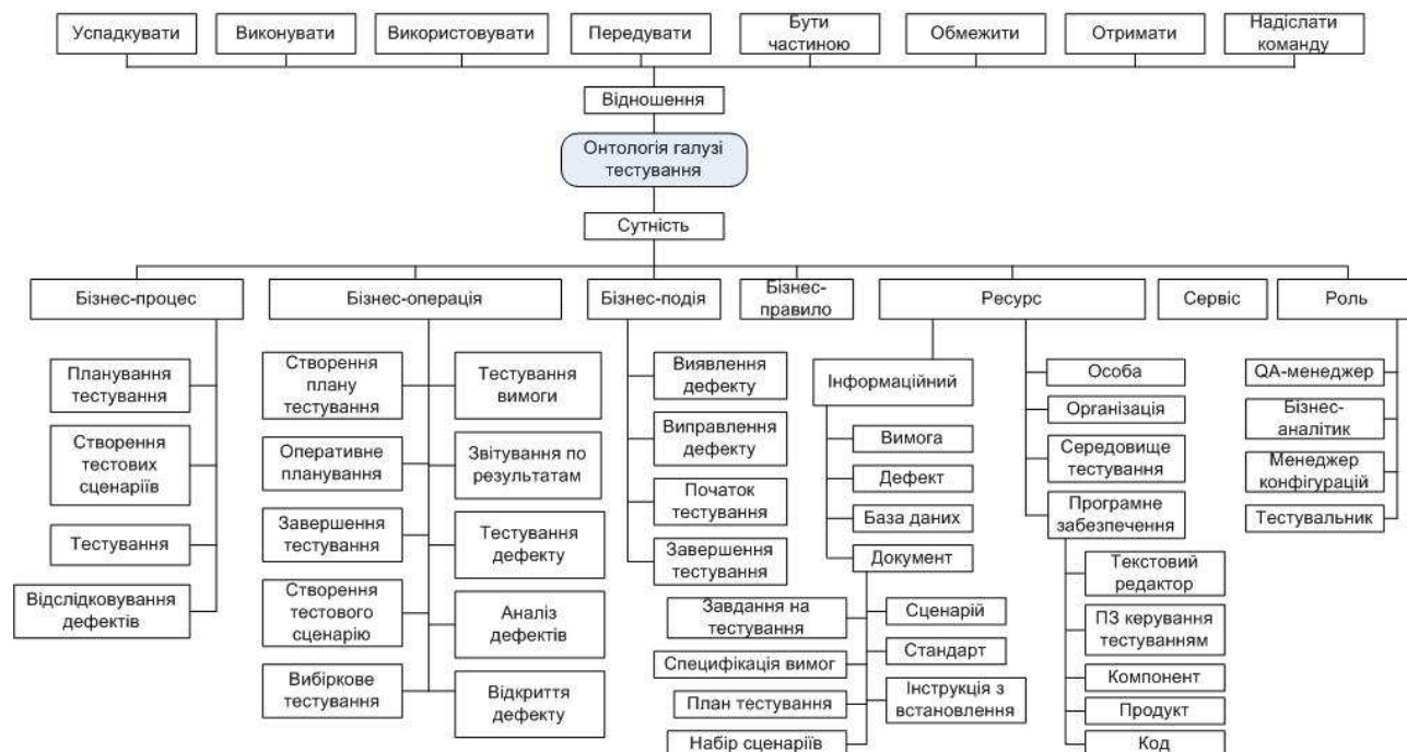
Рис. 7. Сутності та відношення онтології тестування програмного забезпечення
