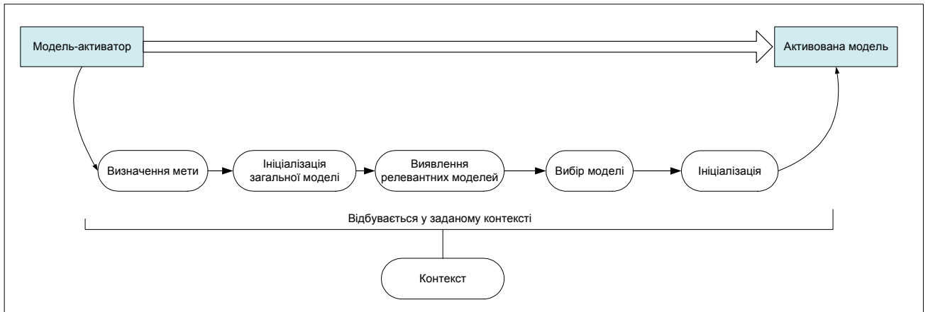
Рис. 3. Процес активації моделі задачі
