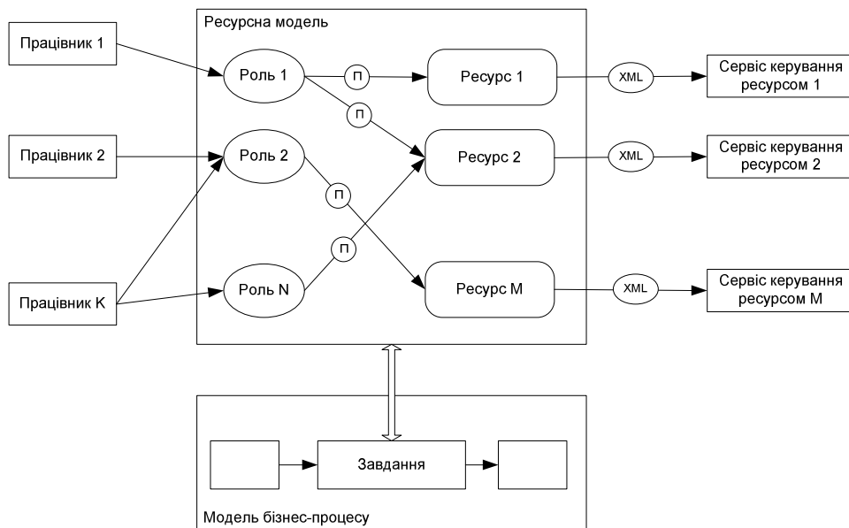
Рис. 8. Структура моделі керування доступом до ресурсів у програмній системі
