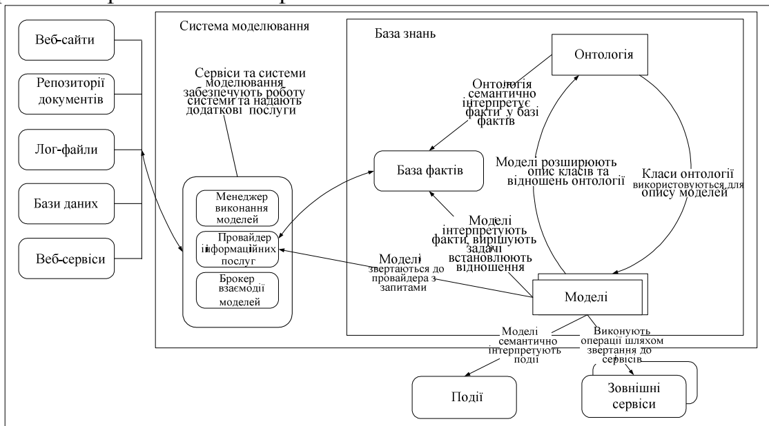
Рис. 2. Структура програмної системи онтологічного моделювання задач
