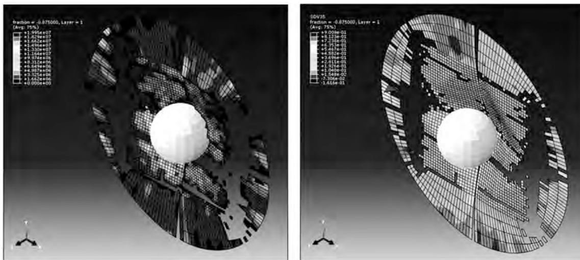
Рис. 6. Ізополя параметру пошкодження у площині пластини із еластичного сіткозміцненого ламінату у критичному діапазоні швидкостей удару: a – ймовірнісна модель деформування і пошкодження [19]; б – розроблена модель еластичного сіткозміцненого матеріалу
