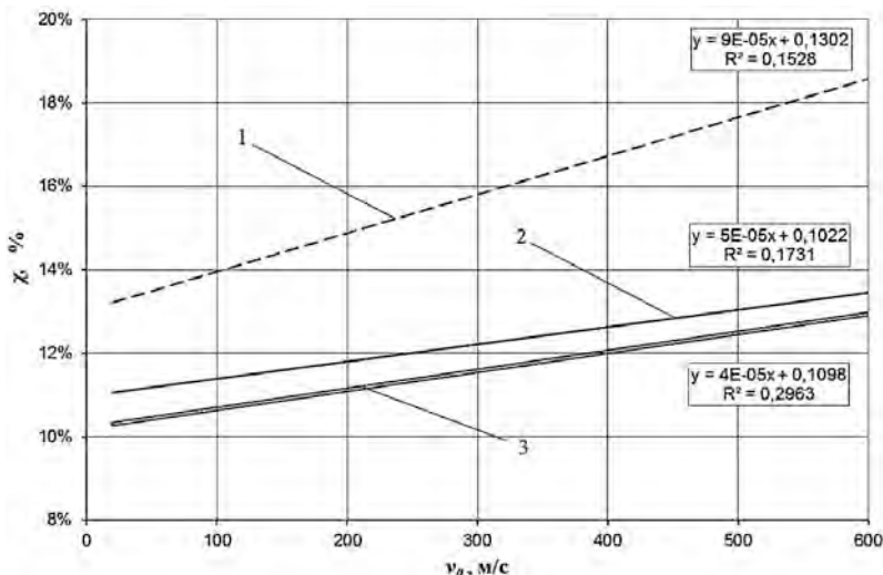
Рис. 3. Залежність похибки розрахунку залишкової енергії ударника від початкової швидкості удару: 1 – стандартна модель волоконнозміцненого матеріалу; 2 – ймовірнісна модель деформування і пошкодження; 3 – розроблена модель еластичного сіткостміцненого матеріалу
