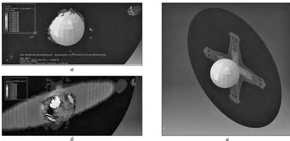
Рис. 4. Етапи адаптації моделі волоконнозміцненого матеріалу для еластичних сіткостміцнених матеріалів: а – стандартна модель волоконнозміцненого матеріалу; б – моделювання двоступінчатого характеру сприйняття навантаження еластичними композитами; в – моделювання сумісної роботи взаємно перпендикулярних ниток волоконного армування
