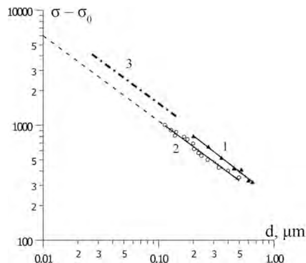
Рис. 12. Структурная чувствительность параметров упрочнения в материалах со сверхмелким зерном: 1 – экструзия; 2 – РКУП; 3 – после протягивания
