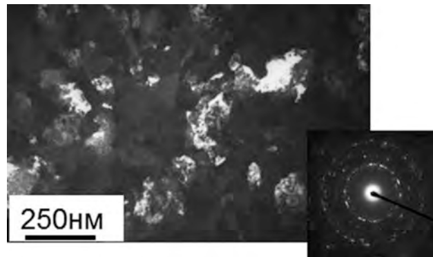
Рис. 9. Структура приповерхностного слоя шара из сплава ВТ-1.0, обработанного накаткой
