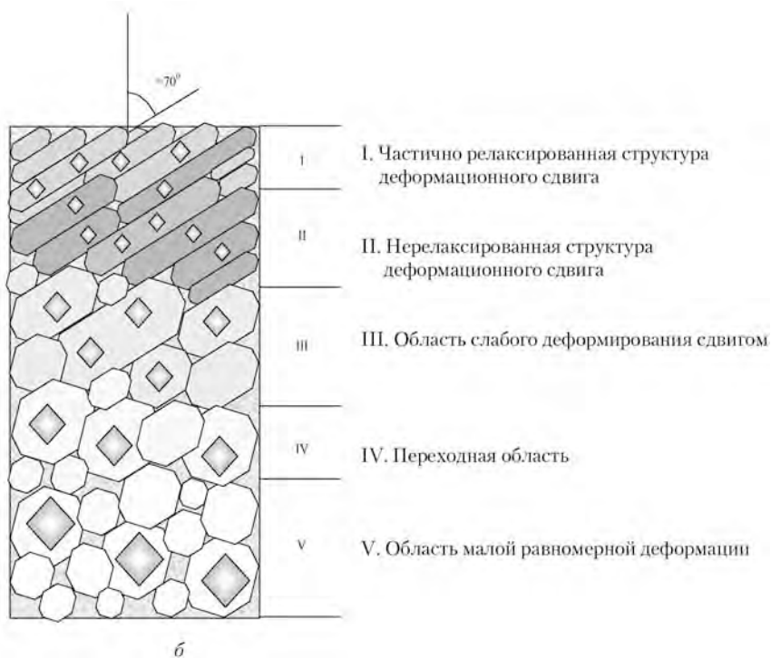
Рис. 2. Структура (а) и схема (б) расположения деформированных слоев
