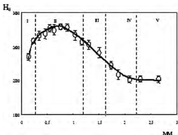
Рис. 4. Зависимость твердости от расстояния до свободной поверхности в протянутых образцах железа
