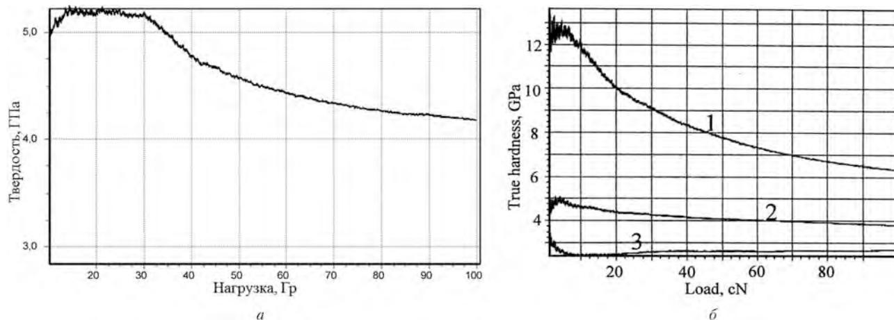
Рис. 10. Изменение микротвердости при непрерывном нагружении в приповерхностном слое титанового сплава ВТ1-0 (а) и стали 65Г (б): 1 – приповерхностный слой; 2 – твердость на глубине 200 мкм.; 3 – твердость в центре образца
