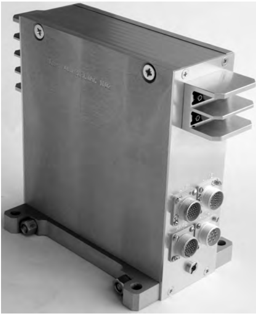
Рис. 1. Зовнішній вигляд центрального блока та резервованого ПМ у складі АГЧ
