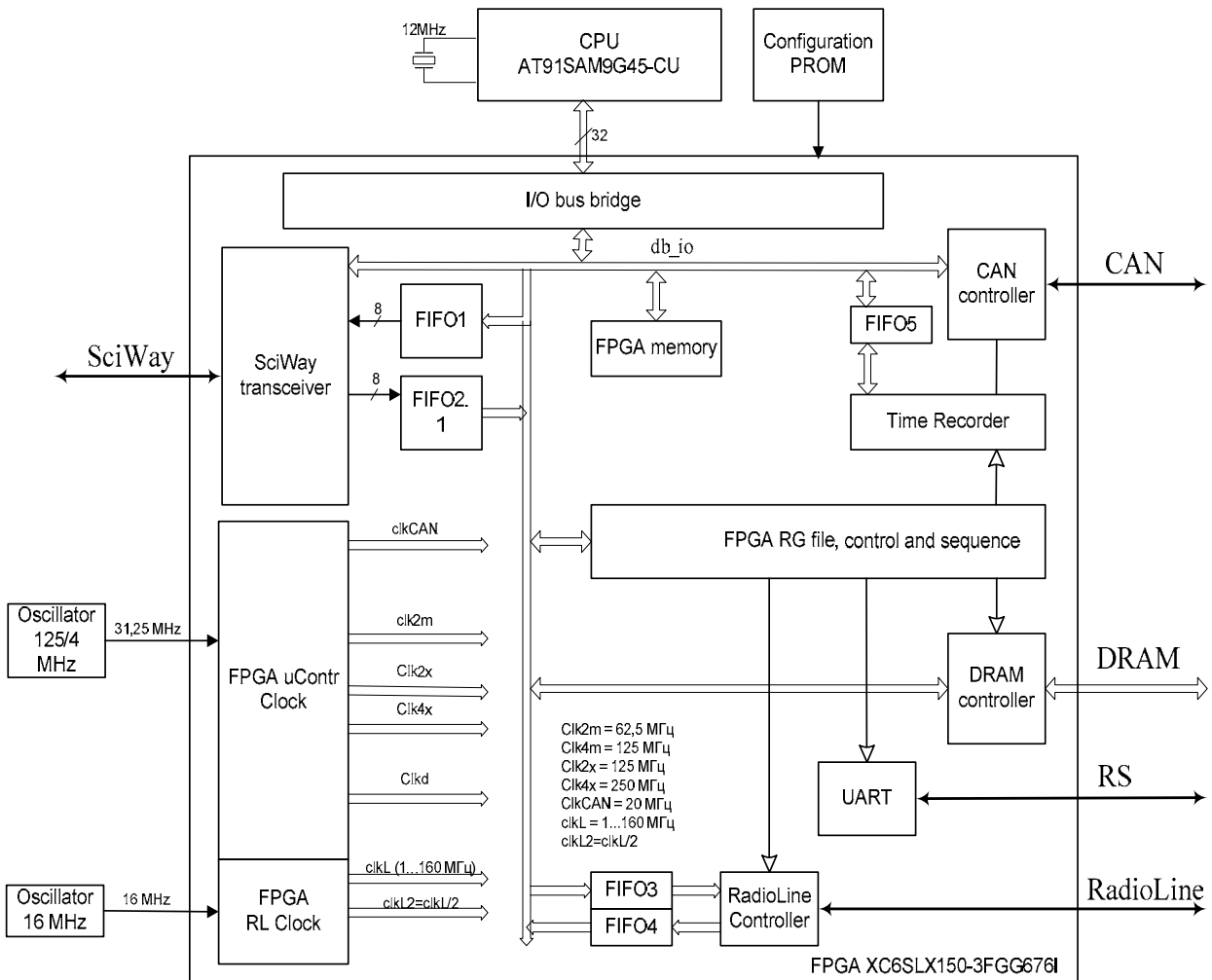
Рис. 2. ПЛІС центрального блока СЗНІ
