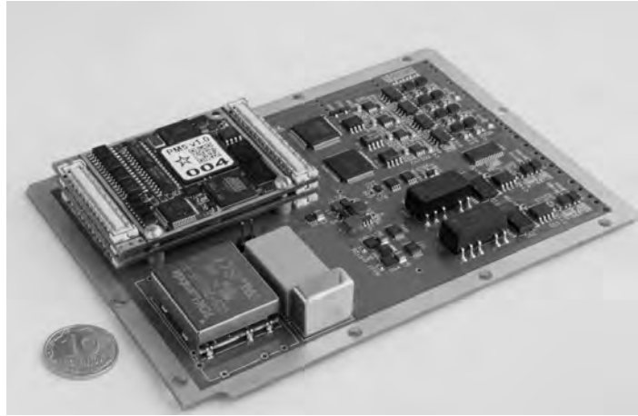
Рис. 1. Зовнішній вигляд центрального блока та резервованого ПМ у складі АГЧ
