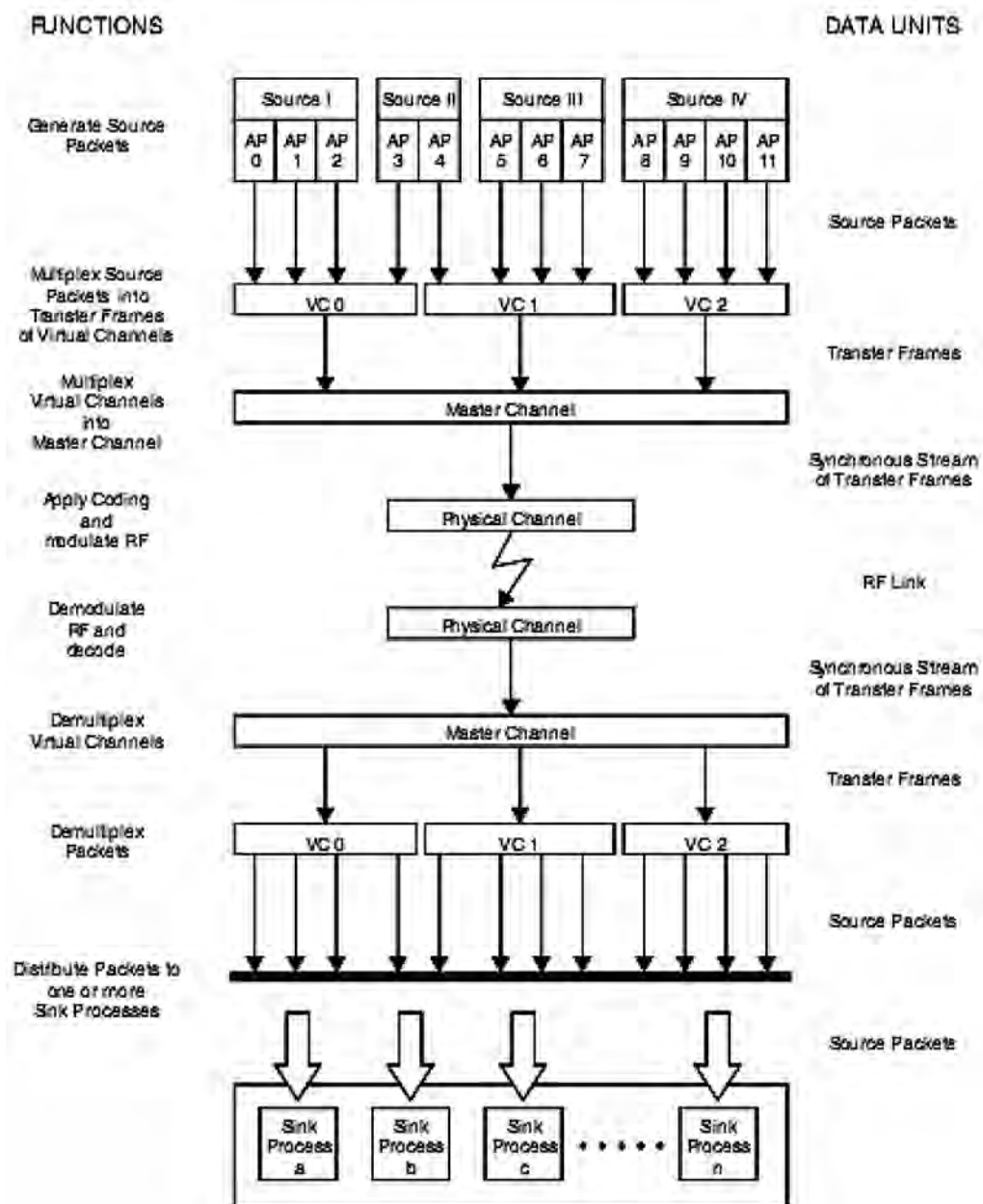
Рис. 3. Модулі СЗНІ у структурі передачі телеметричної інформації
