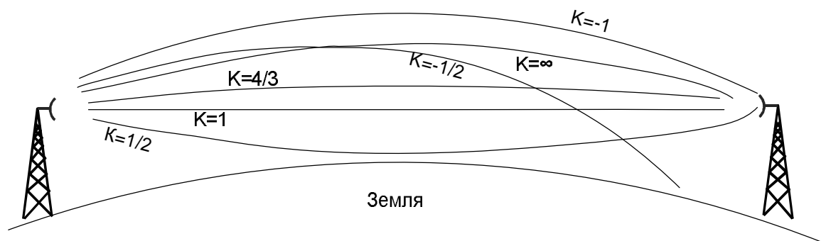
Рис. 1. Умови поширення радіохвиль залежно від К-фактора
