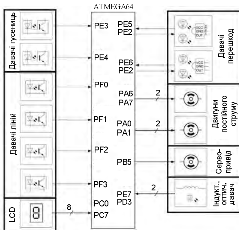
Рис. 2. Структурна схема стенда
