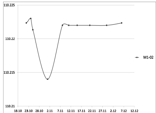
Рис. 10. График просадки по марке, м
