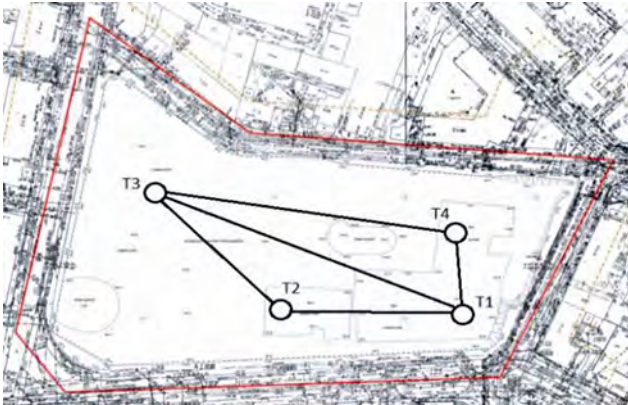
Рис. 5. Схема внутренней опорной сети
