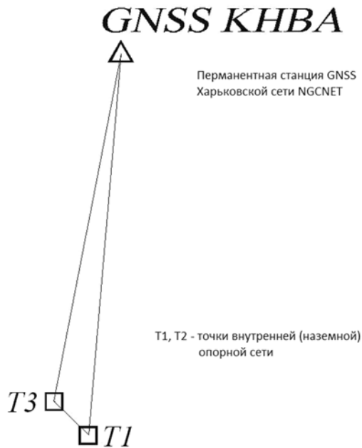
Рис. 4. Схема привязки базовых точек
