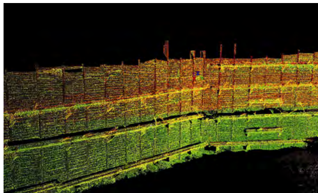
Рис. 1. Модель подпорной стены в виде облака точек
