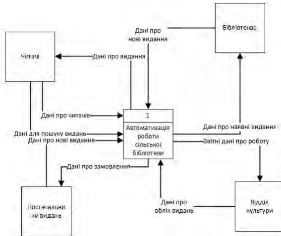
Рис. 1. Контекстна діаграма потоків даних бібліотечного фонду
