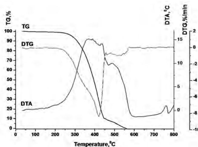
Рис. 1. Термограма зразка залишкової оливи
