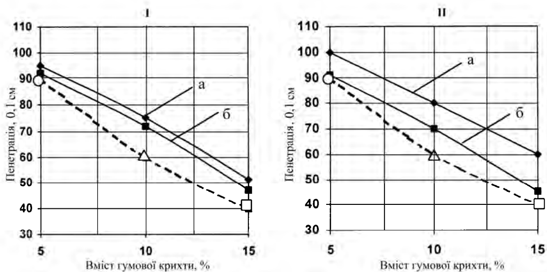
Рис. 1. Зміна пенетрації для ГБВ залежно від вмісту гумової крихти для умов: (I) – тривалість змішування 250 хв., температура T = 433\text{ K} ; (II) – тривалість змішування 350 хв., температура T = 433\text{ K} ; (а) – ГК \varnothing 0,6\div 0,8\text{ мм} ; (б) – ГК \varnothing 0,8\div 1\text{ мм} ; О – БПВ 90; \Delta – БПВ 60; \square – БПВ 40
