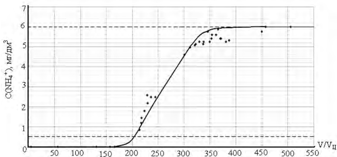
Рис. 2. Залежність концентрації \text{NH}_4^+ у фільтраті від об'єму розчину, що пройшов крізь колонку з цеолітокерамічним адсорбентом
