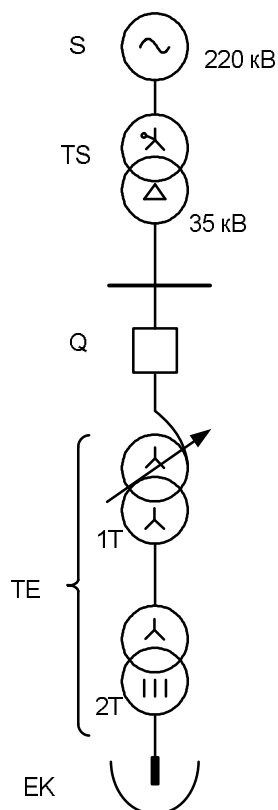
Рис. 1. Система електропостачання дугової сталетопної печі:
