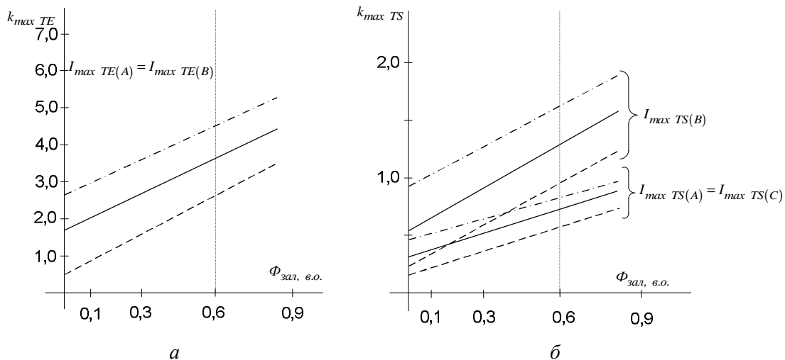
Рис. 2. Залежності кратності КСН від величини залишкового потоку магнітної системи пічного агрегату:
