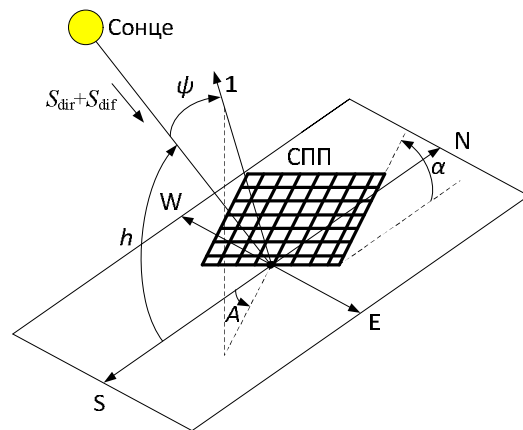
Рис. 2. Параметри орієнтації СПП відносно горизонтальної площини: \alpha – кут нахилу, A – азимут, \gamma – кут падіння, h – кут висоти Сонця
