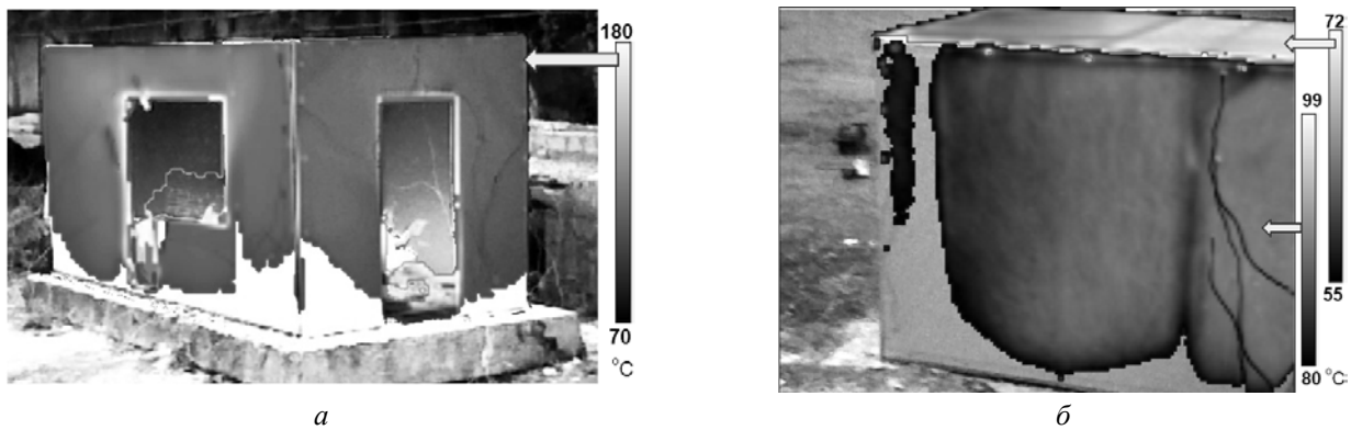
Рис. 3. Нагрів зовнішньої поверхні огорожувальних конструкцій під час пожежі П-D-I ( q_{f,d}=525 \text{ Дж/м}^2 ; t_{max}=18 \text{ хв} ; T_{max}=307 \text{ °C} ): а – фото відповідає 25-й хв експерименту; б – фото відповідає 35-й хв експерименту
