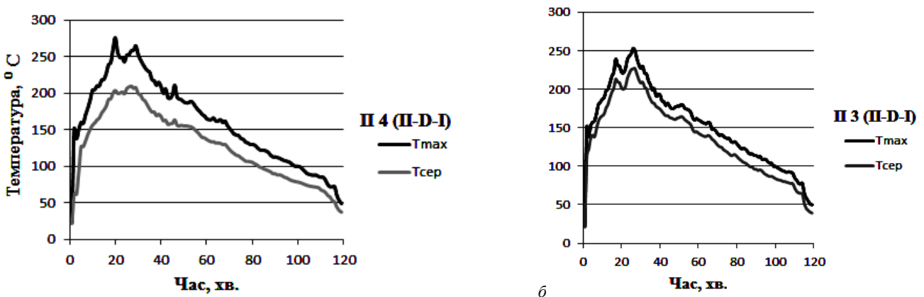
Рис. 2. Залежність температура–час експерименту II-D-I ( q_{f,d}=525 \text{ Дж/м}^2 ; T_{max}=307 \text{ °C} ): а – для стінки з балконом (П4); б – для стінки з дверима (П3)
