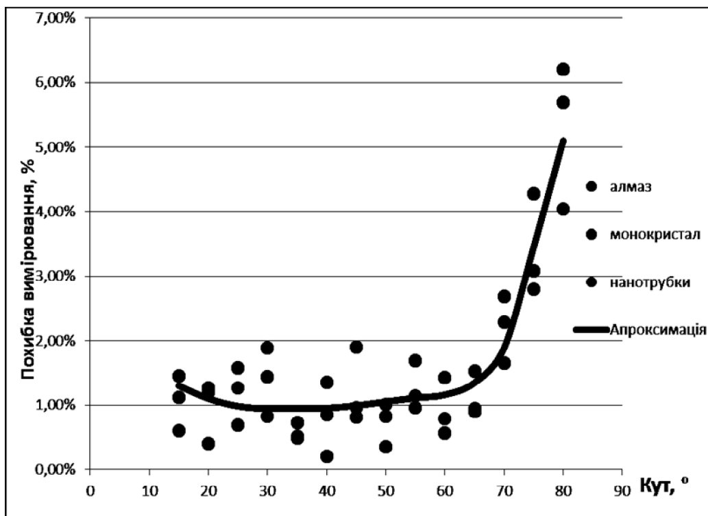
Рис. 2. Залежність точності вимірювання температури від кута між лазером та досліджуванним об'єктом (температура 20^{\circ}\text{C} )
