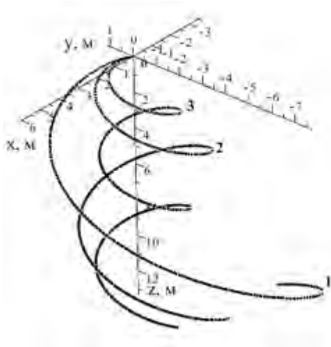
Рис. 2. Три траєкторії для різних \omega_0
