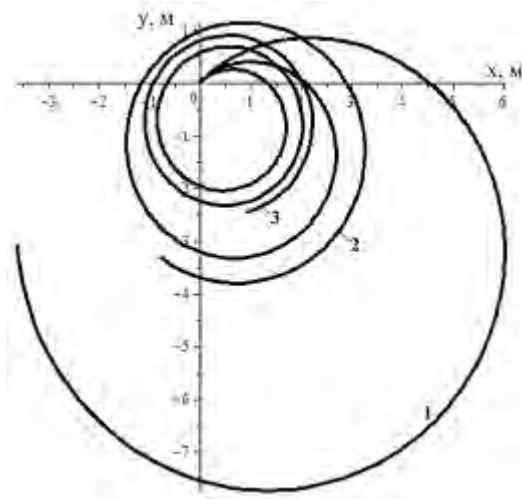
Рис. 3. Проекції траєкторій на площину xoy
