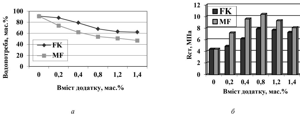
Рис. 1. Вплив добавок FK і MF на водопотребу (а) і міцність (б) гіпсового в'яжучого із фосфогіпсу
